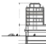
Schnitt MST: 1_2000
