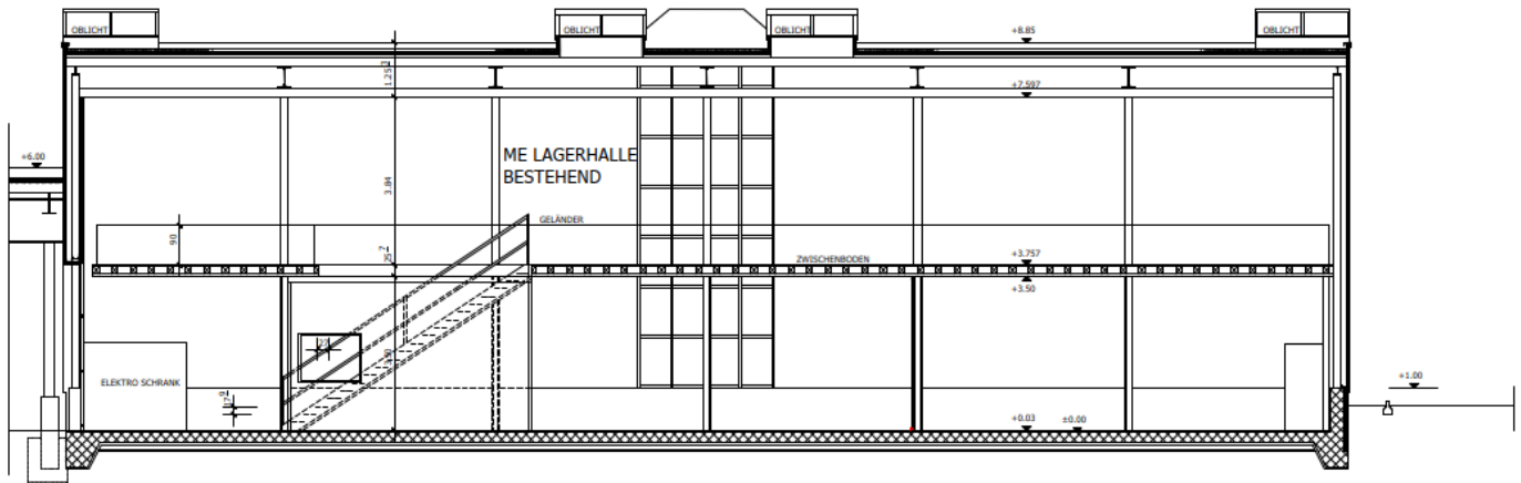
SCHNITT A-A
