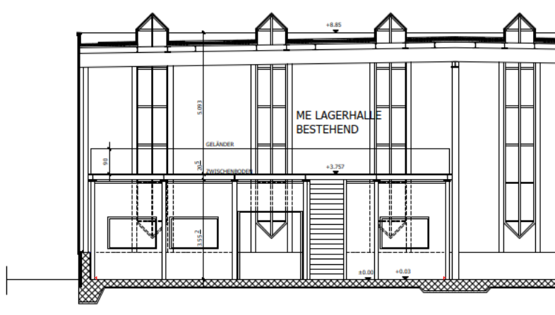
SCHNITT B-B
