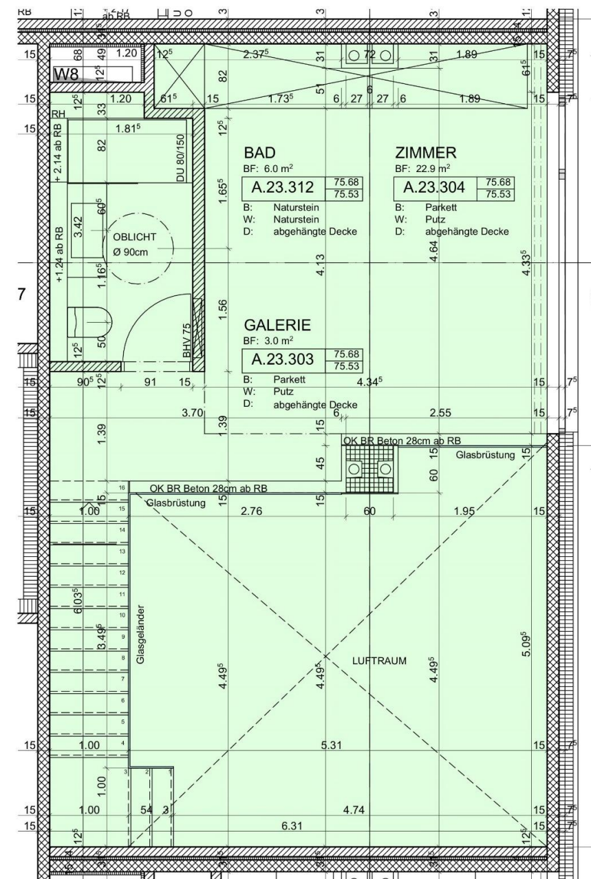
24. Obergeschoss
