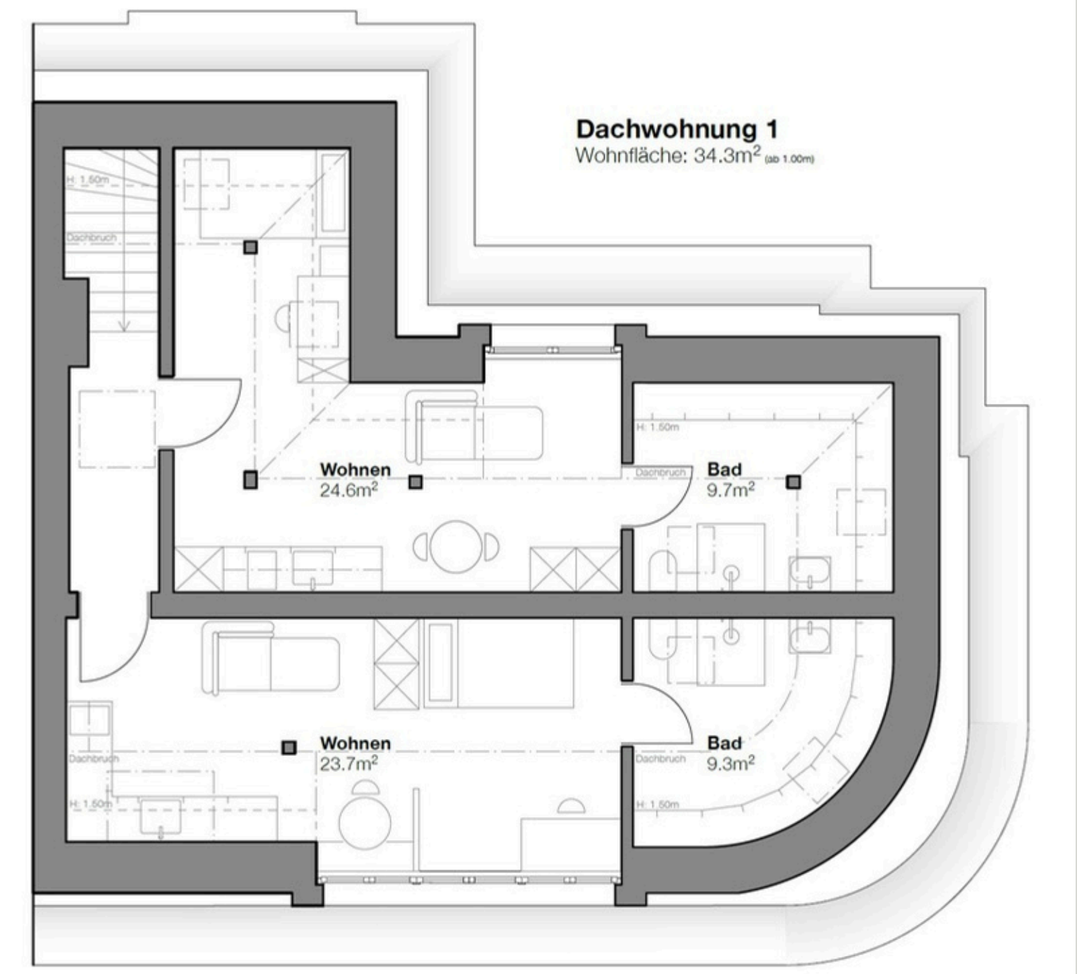
Dachgeschoss
