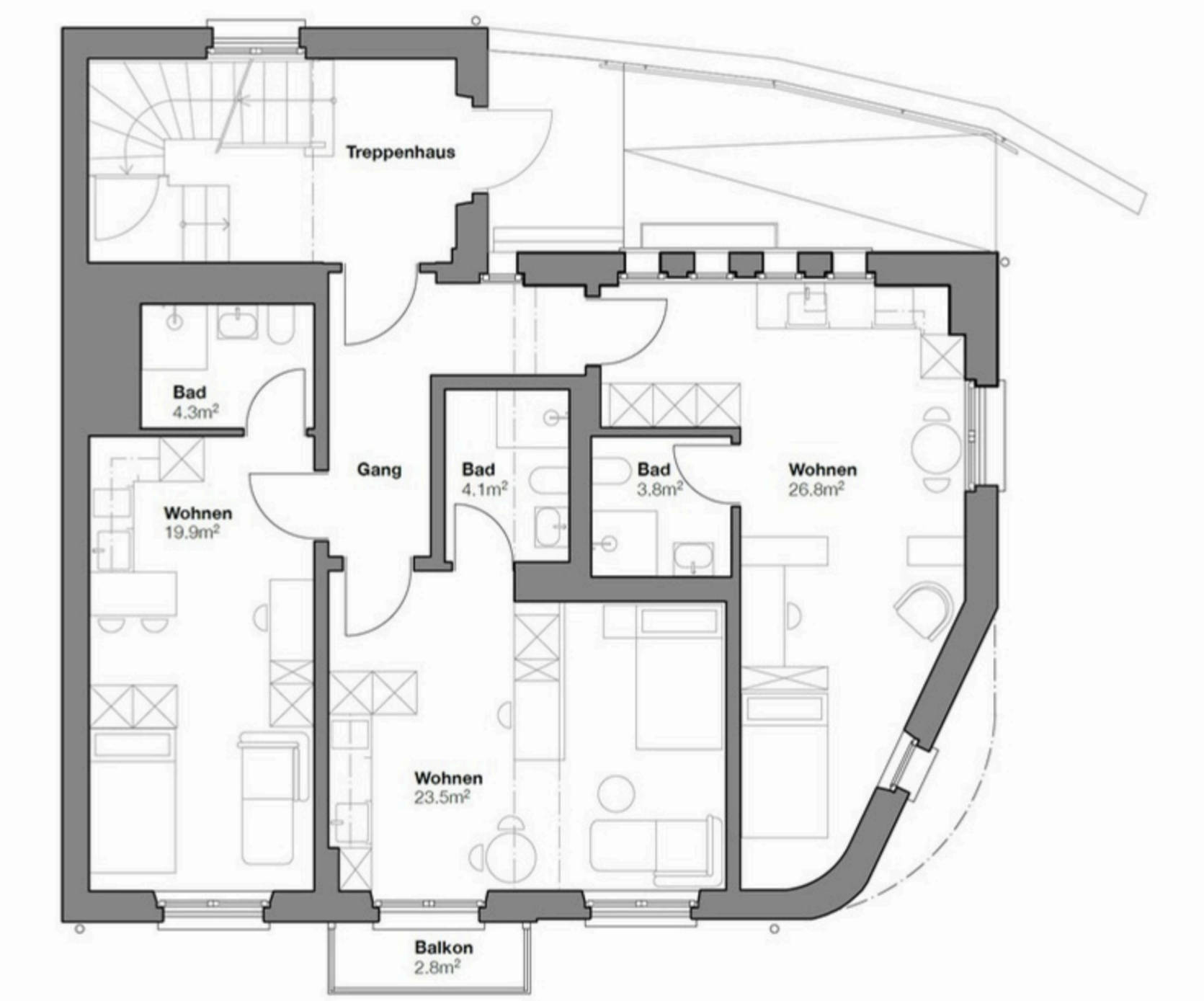
Erdgeschoss
