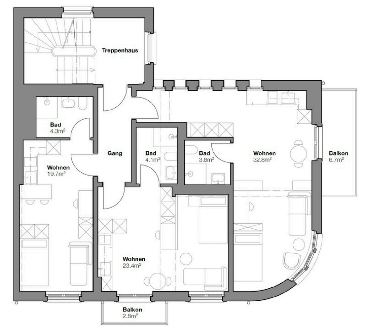
1.Obergeschoss
