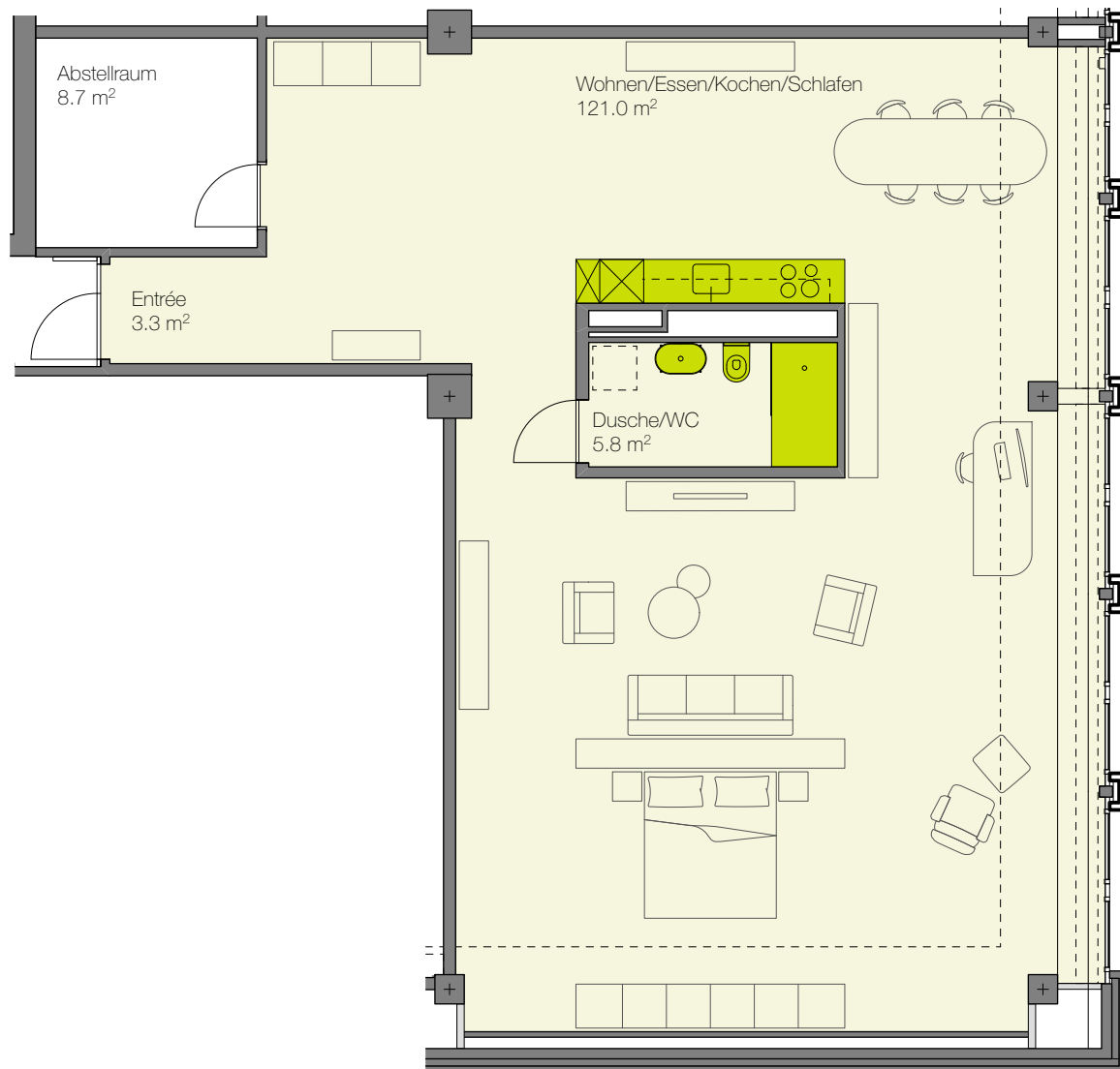
Grundriss 5. Obergeschoss Mst. 1:100
