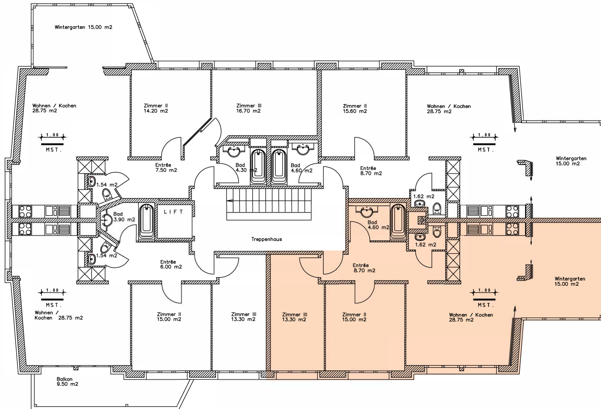
2. Obergeschoss 1:100 Kesselweg 12, 4410 Liestal
