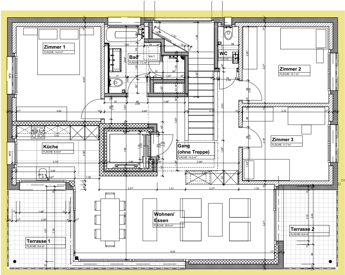
Wohnung C10 Nettowoohnfläche: 105.5 m² Mst. 1:100
