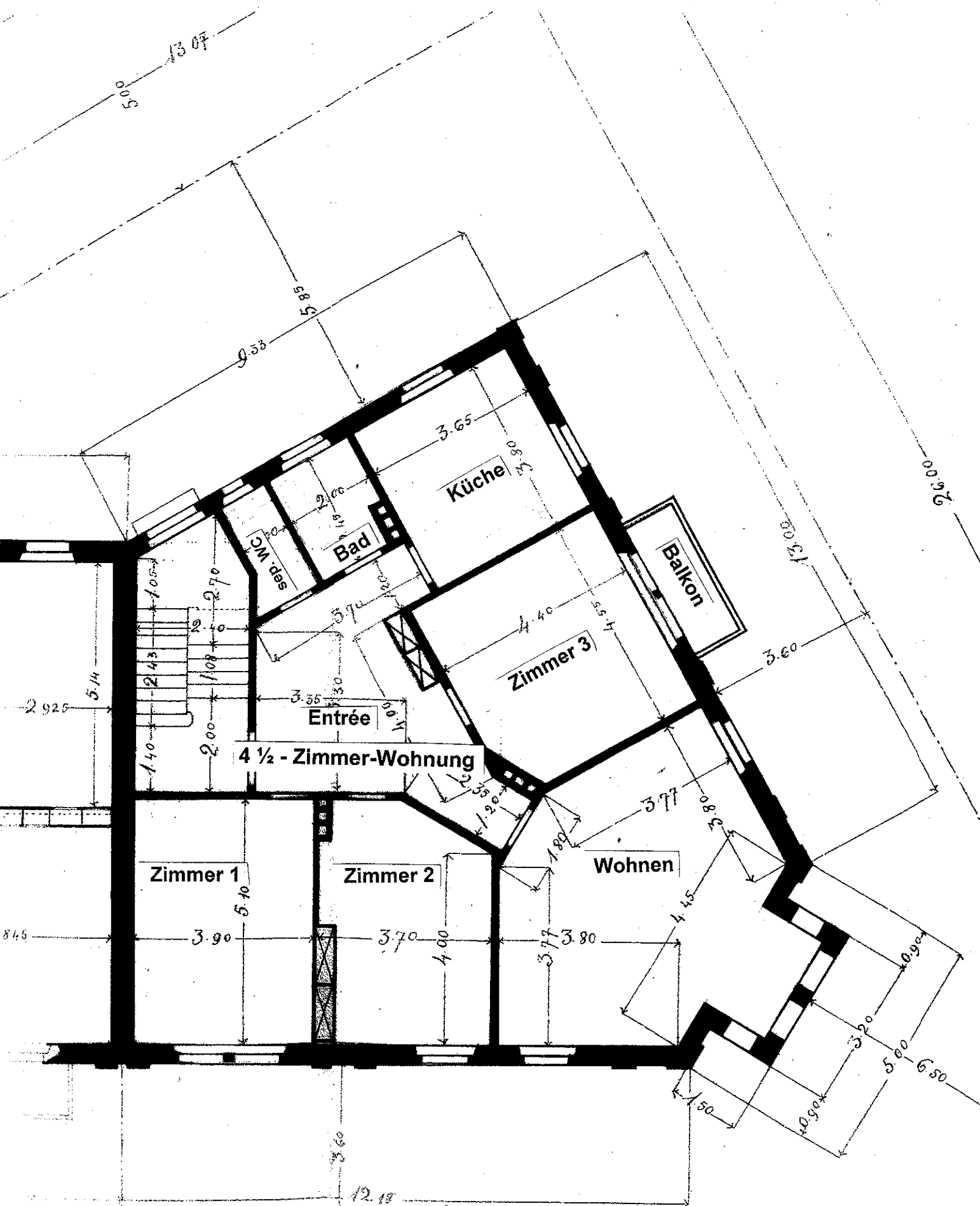
1. OBERGESCHOSS 1 : 100
