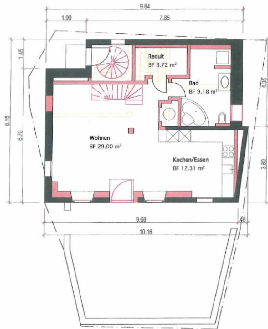
Grundriss UG
