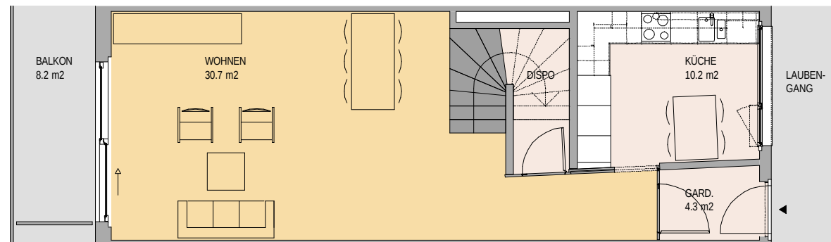
GRUNDRISS 1.OG
