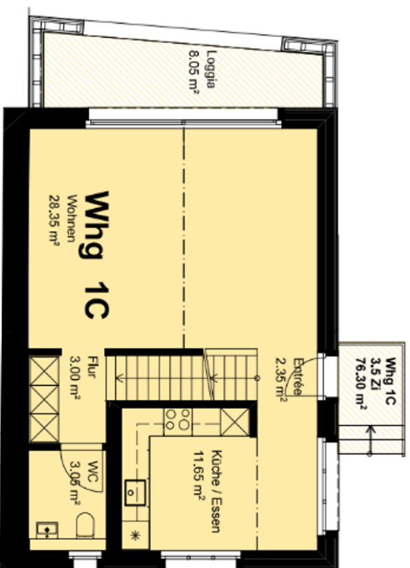
Erdgeschoss
