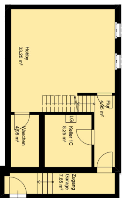
Untergeschoss ( 59.05 m² )
