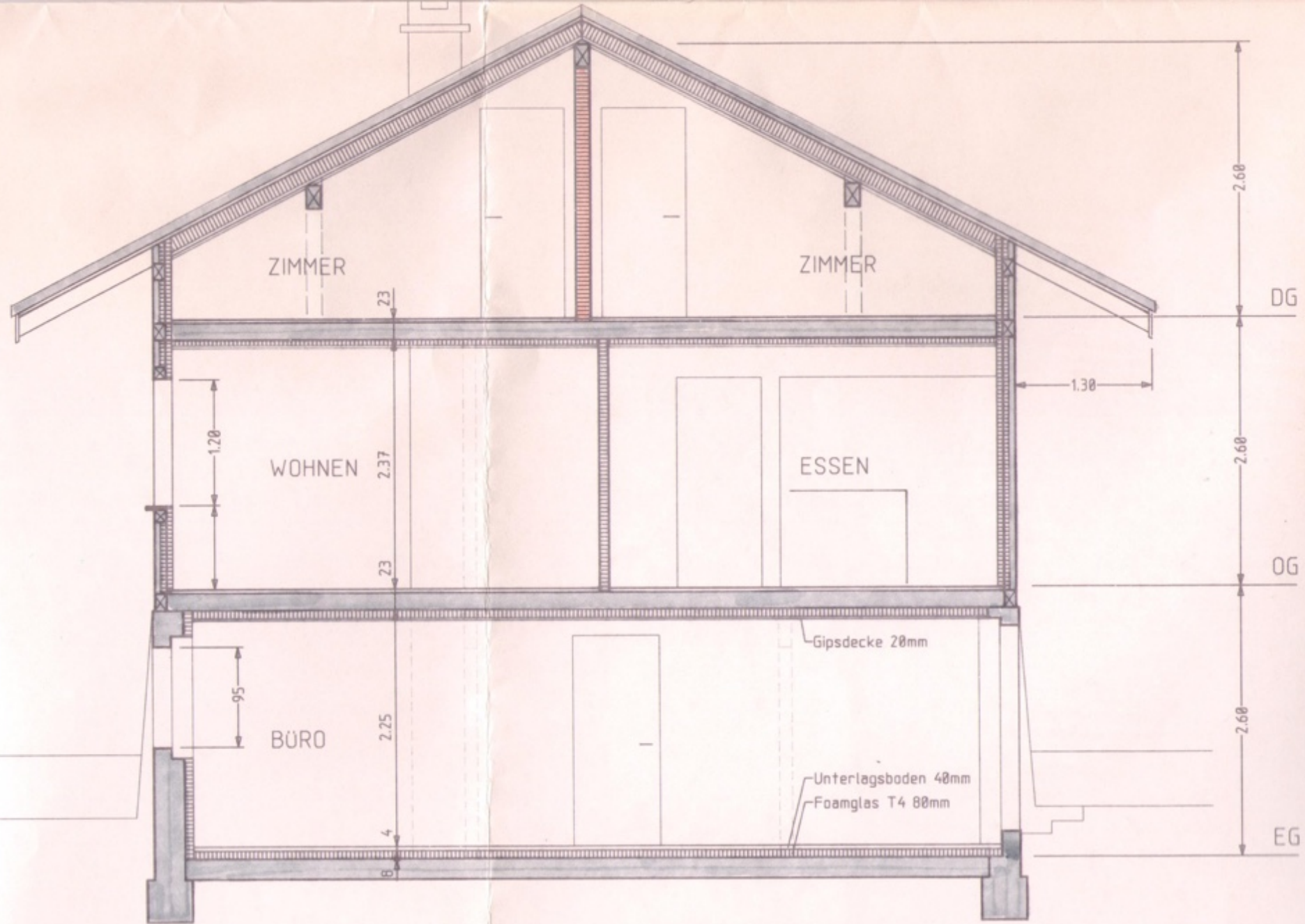
SCHNITT A-A
