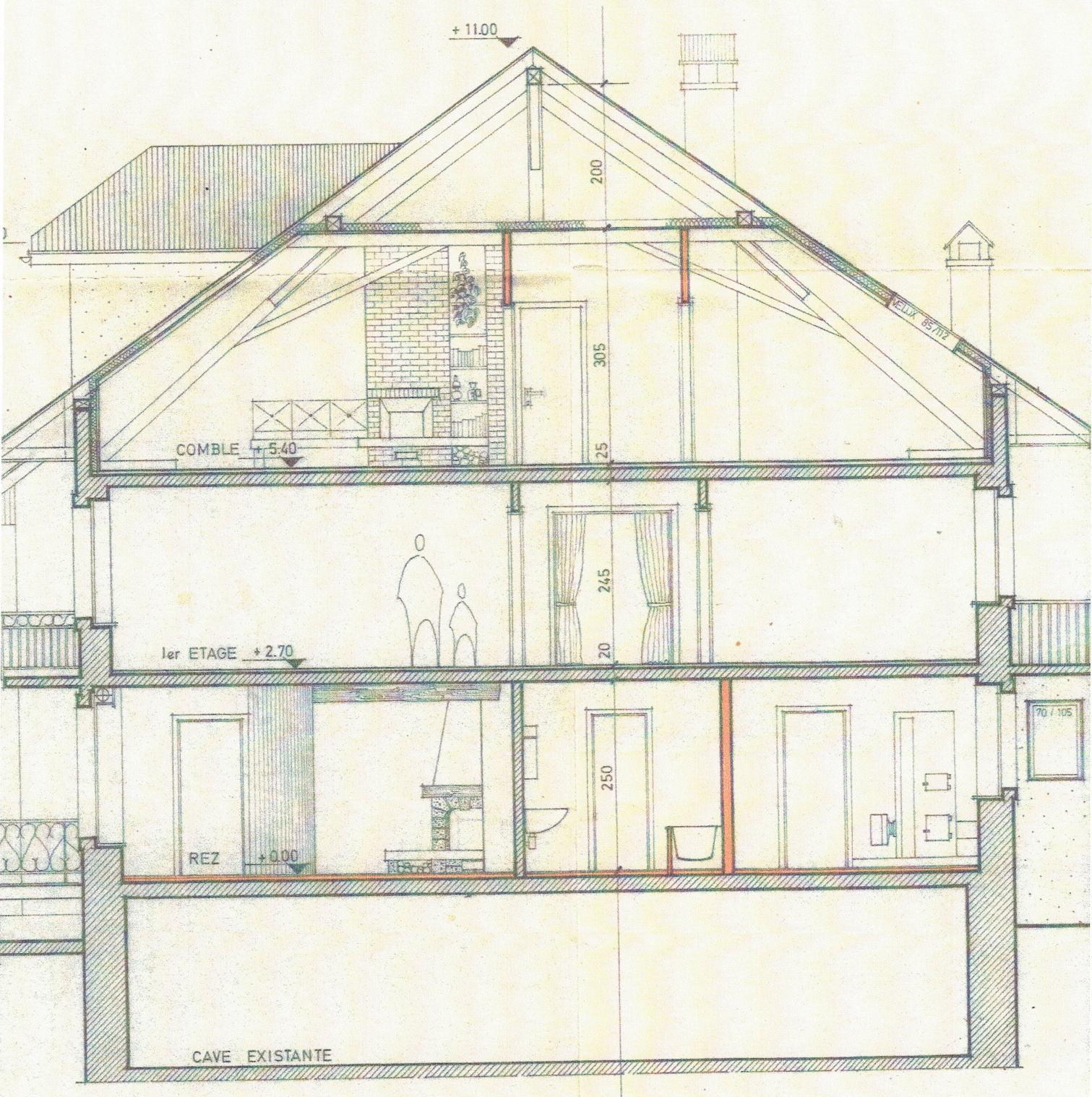
coupe a - a
