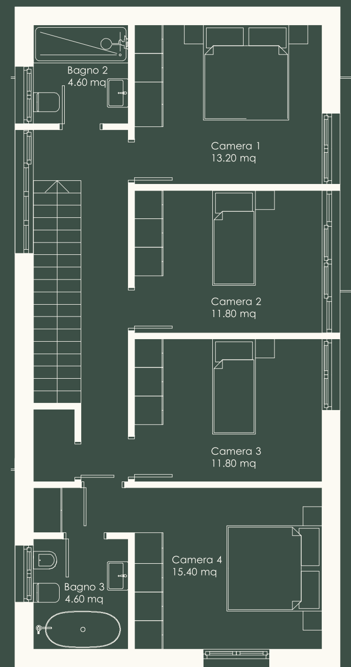
Primo Piano
