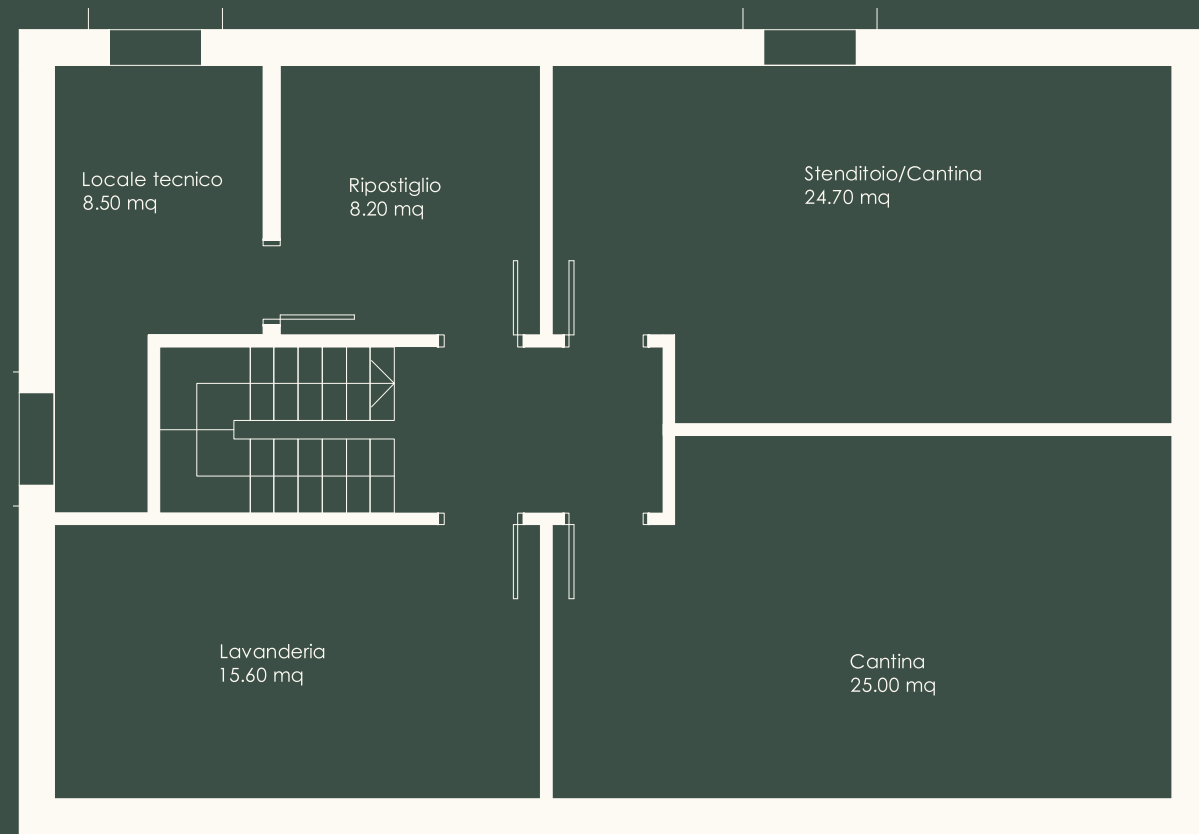
Primo interrato
