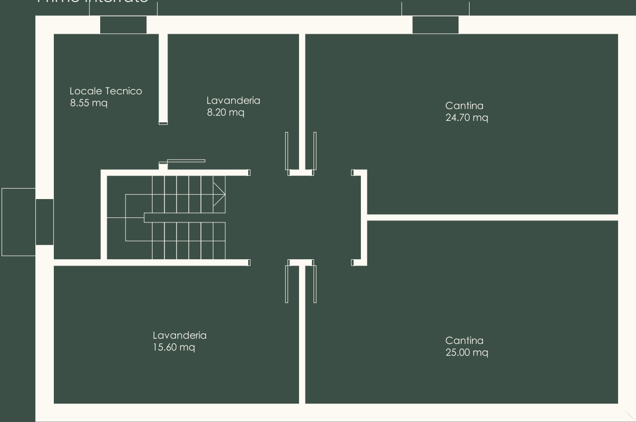
Primo interrato
