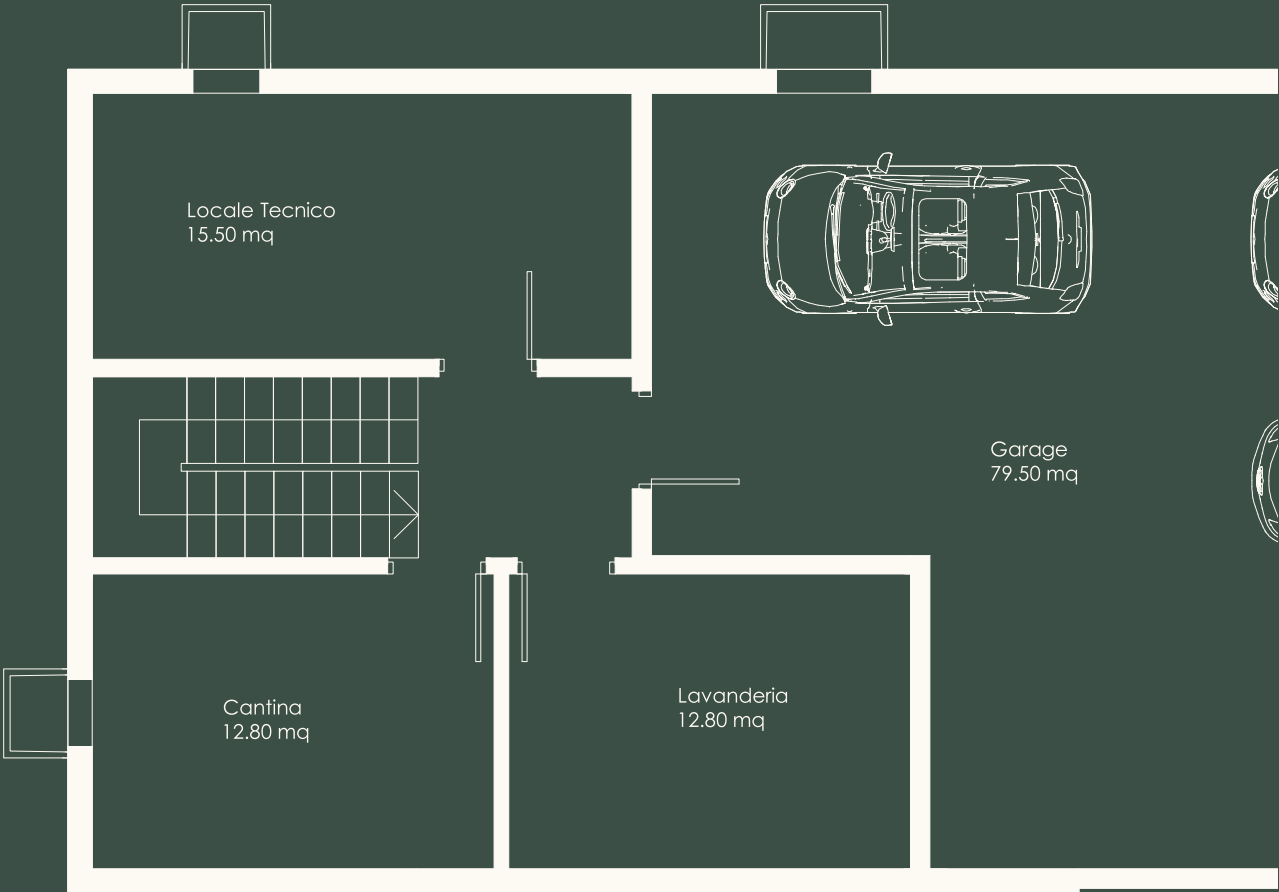
Primo interrato
