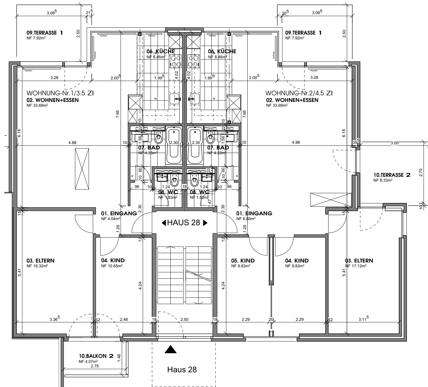
HAUS NR. 28: ERDGESCHOSS
