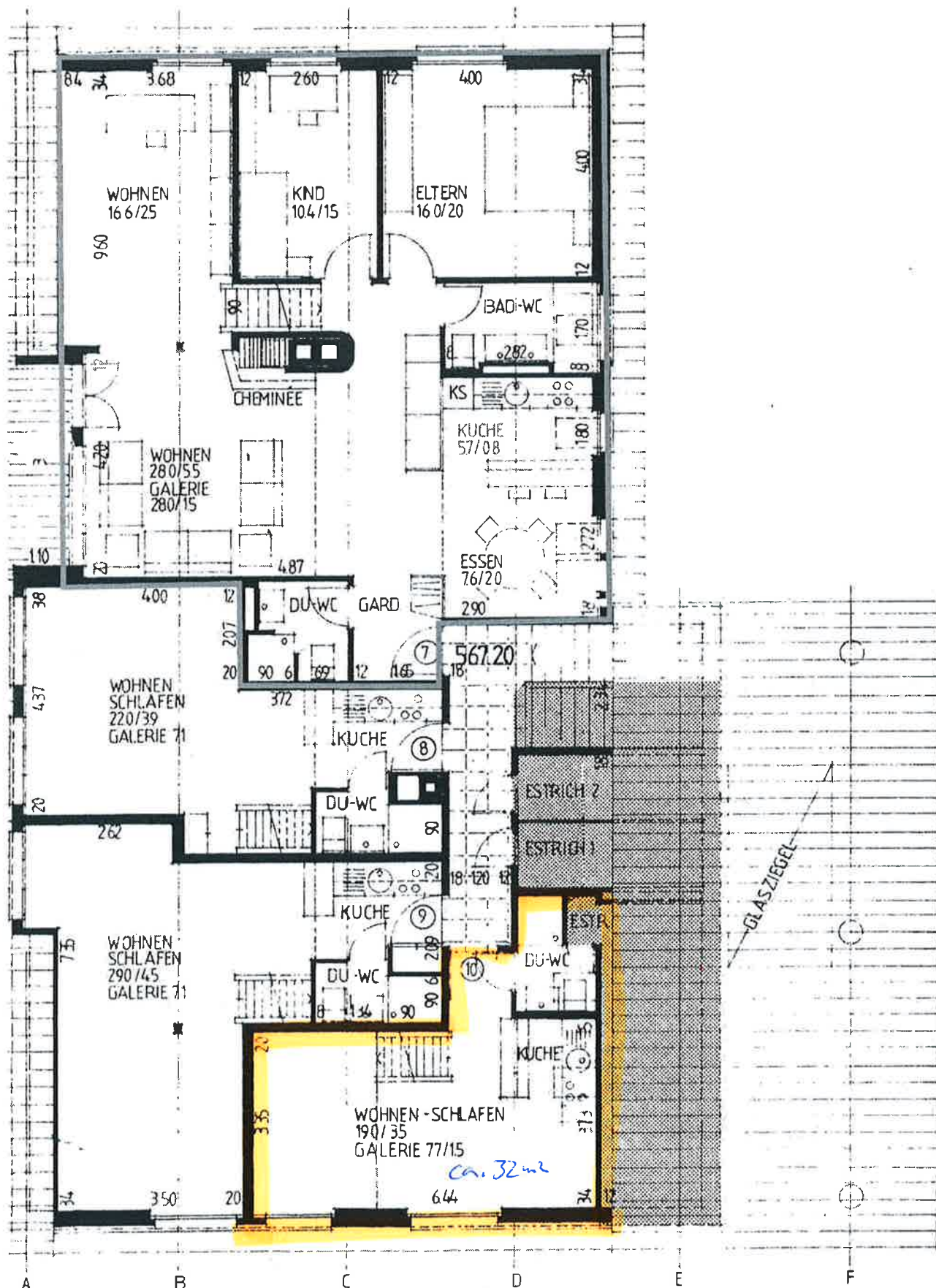
GRUNDRISS DACHGESCHOSS
