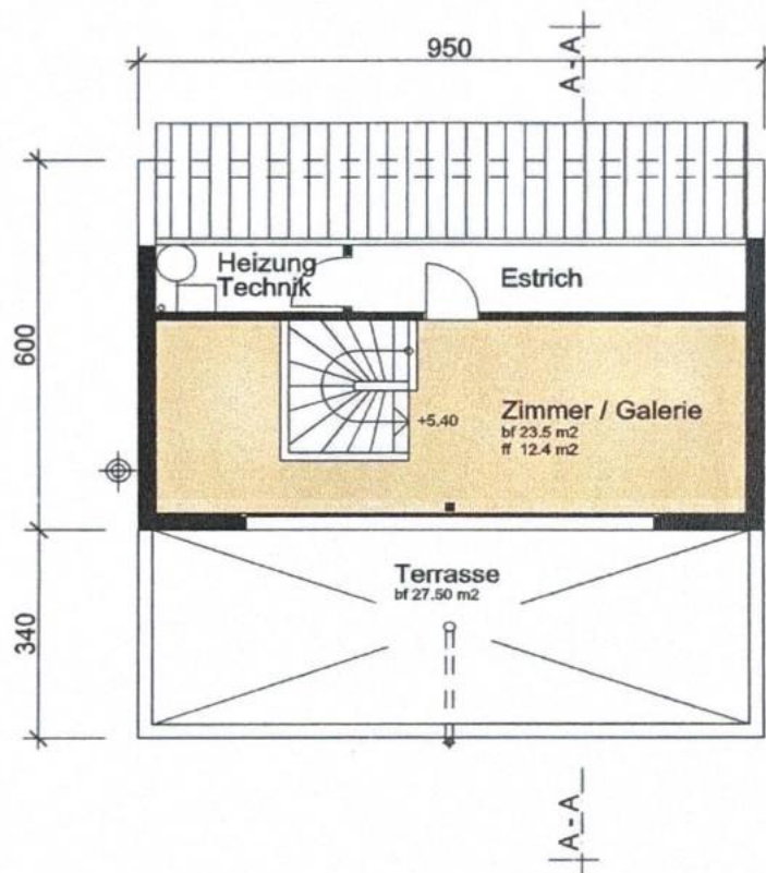
Haus C6 Dachgeschoss
