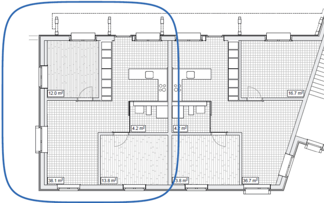
Erdgeschoss 1:100
