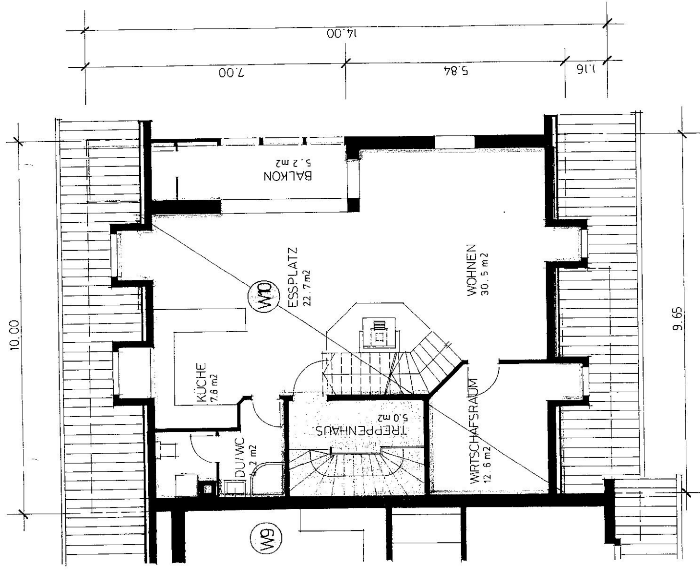
GRUNDRISS 2. OBERGESCHOSS MST. 1:100
