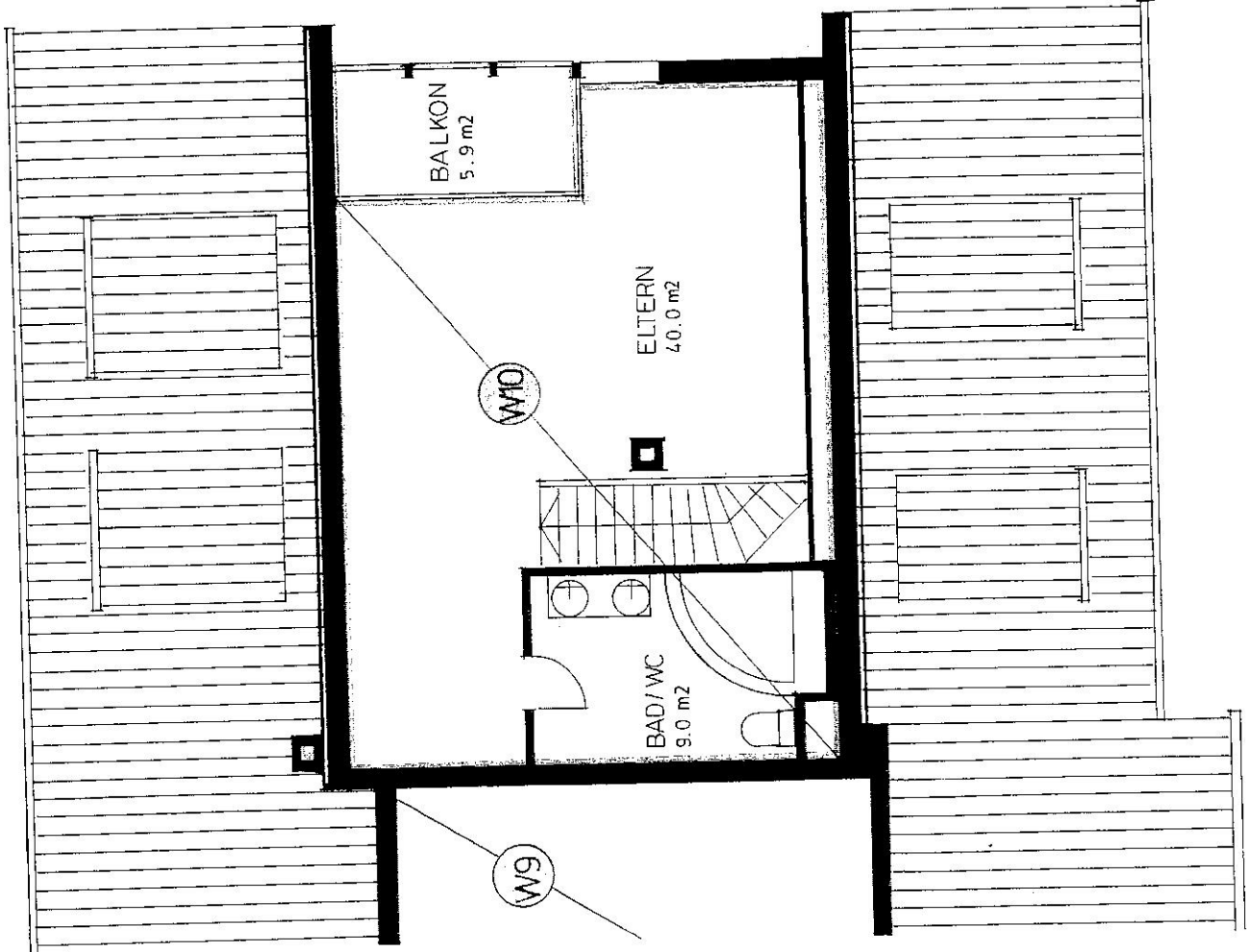
GRUNDRISS DACHGESCHOSS MST. 1 : 100
