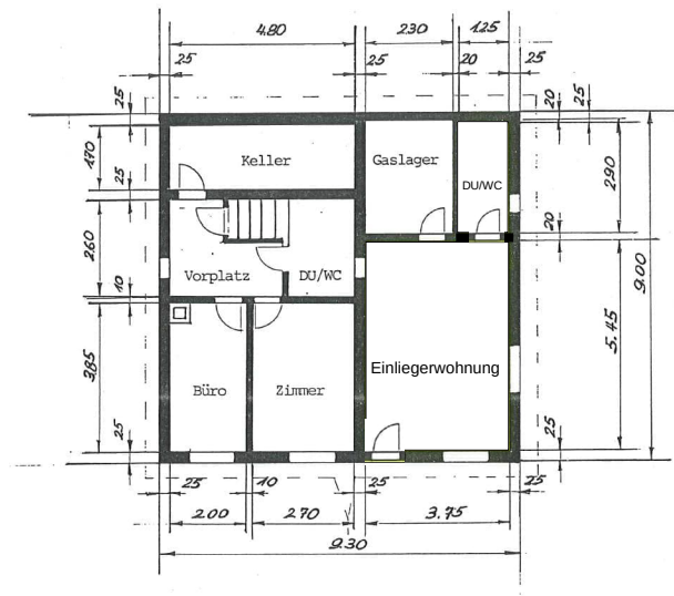
Grundriss Erdgeschoss
