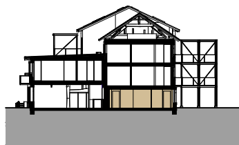
Schnitt
