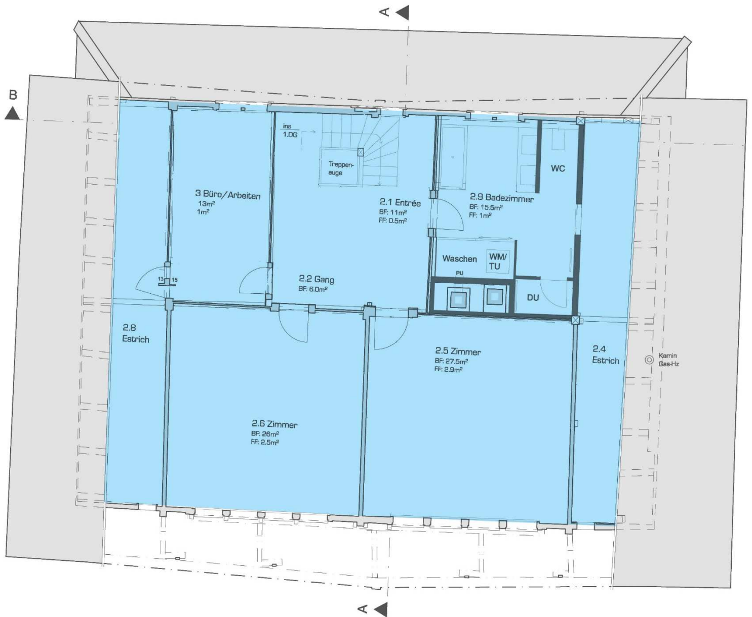
2. Obergeschoss
