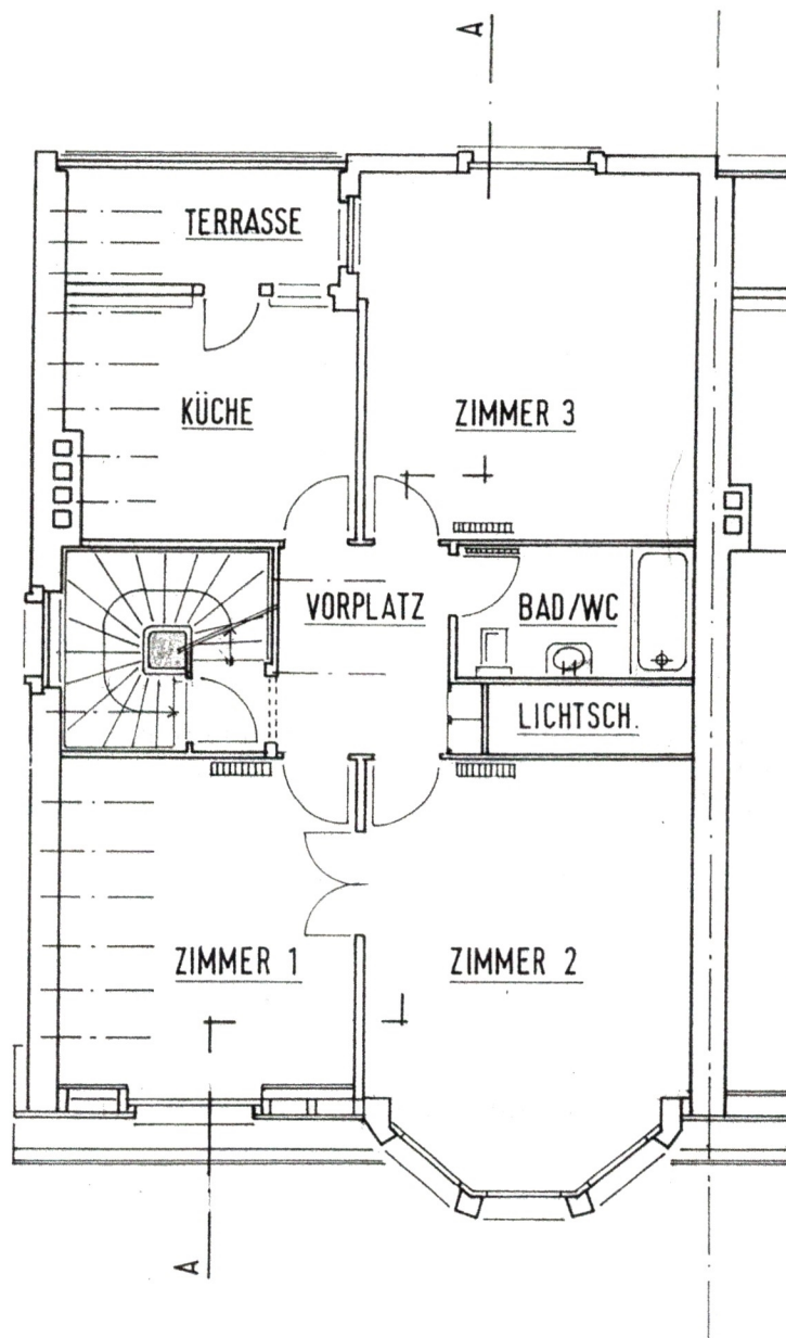
GRUNDRISS 3.06
