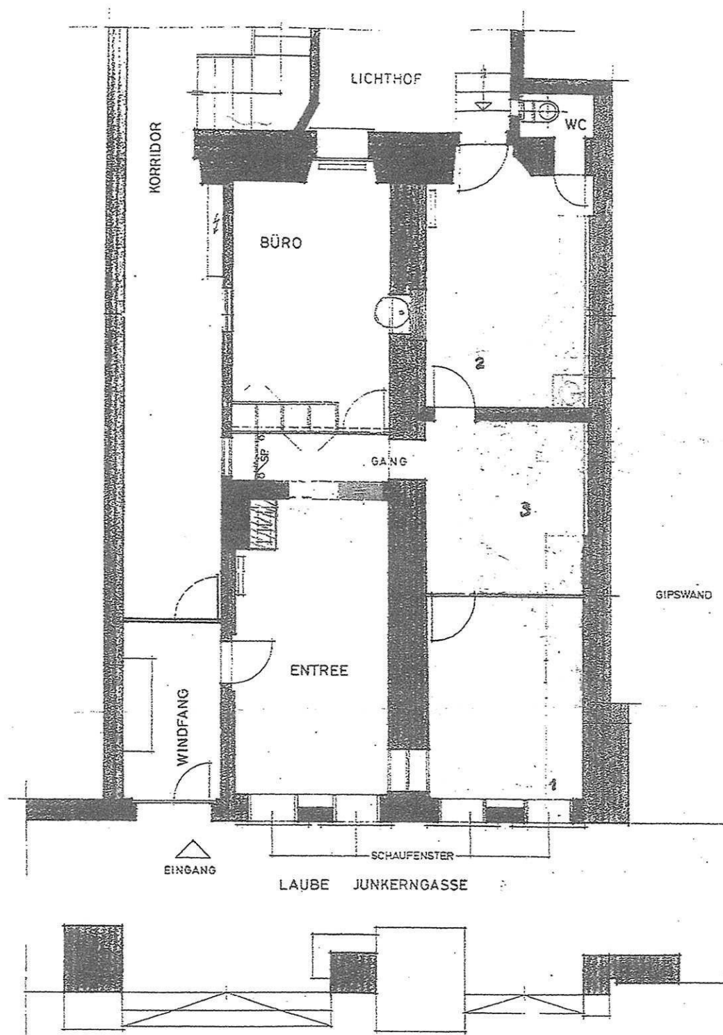
GRUNDRISS MST, 1:100
