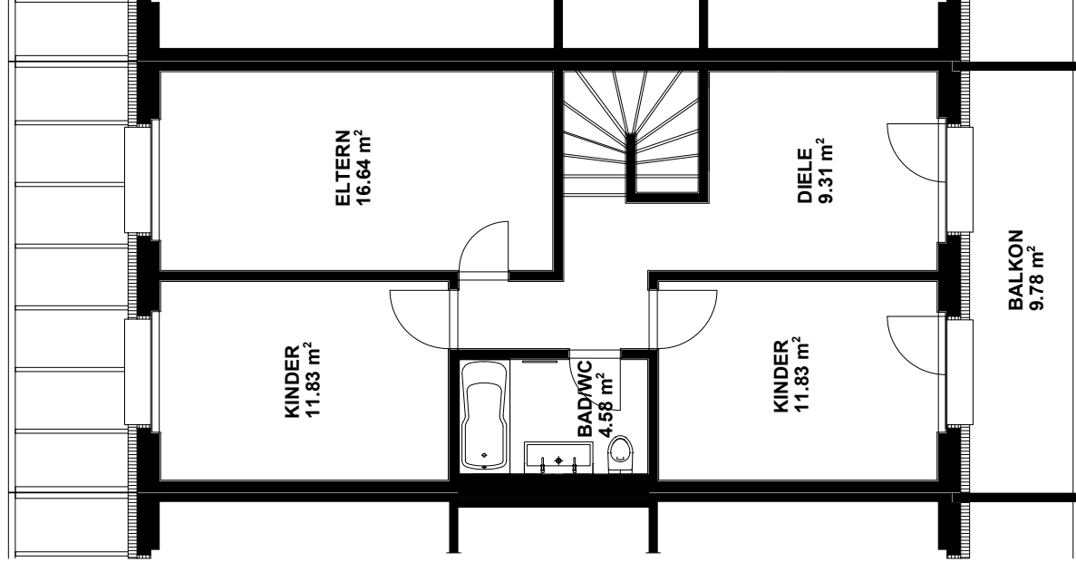
Obergeschoss 1:100
