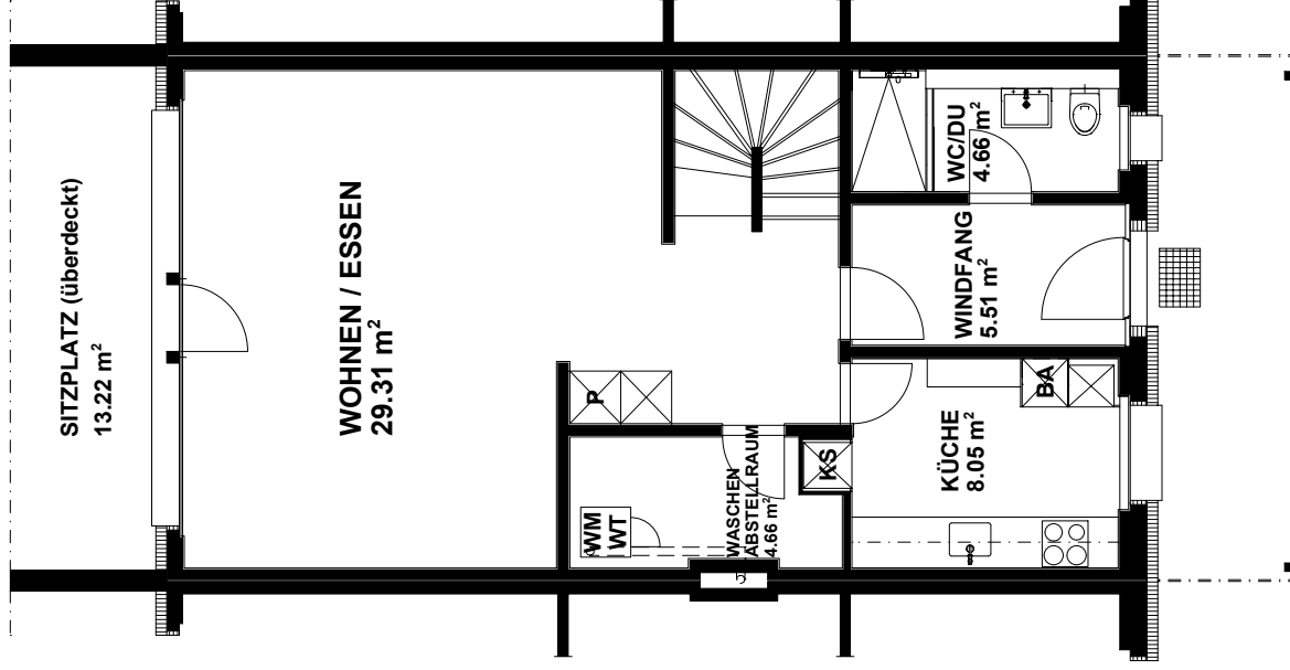
Erdgeschoss 1:100
