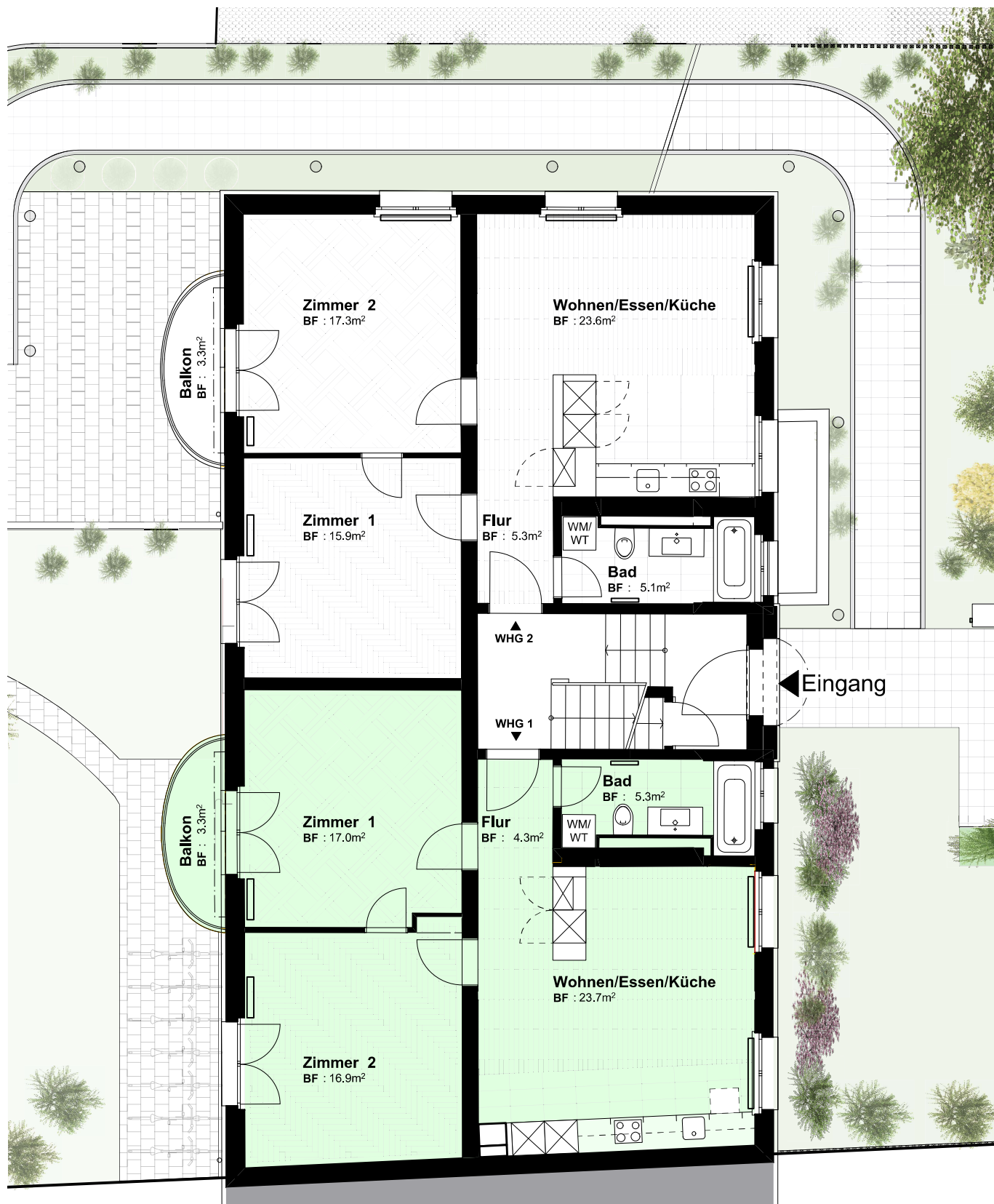
Erdgeschoss
