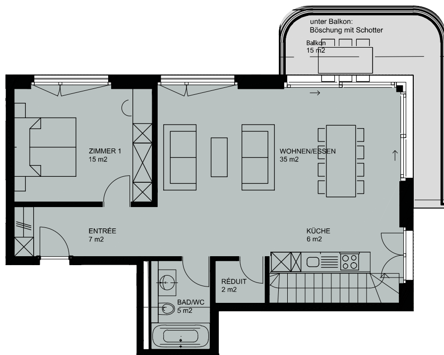
Erdgeschoss
