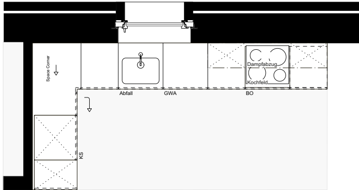
Küche Mst. 1:50
