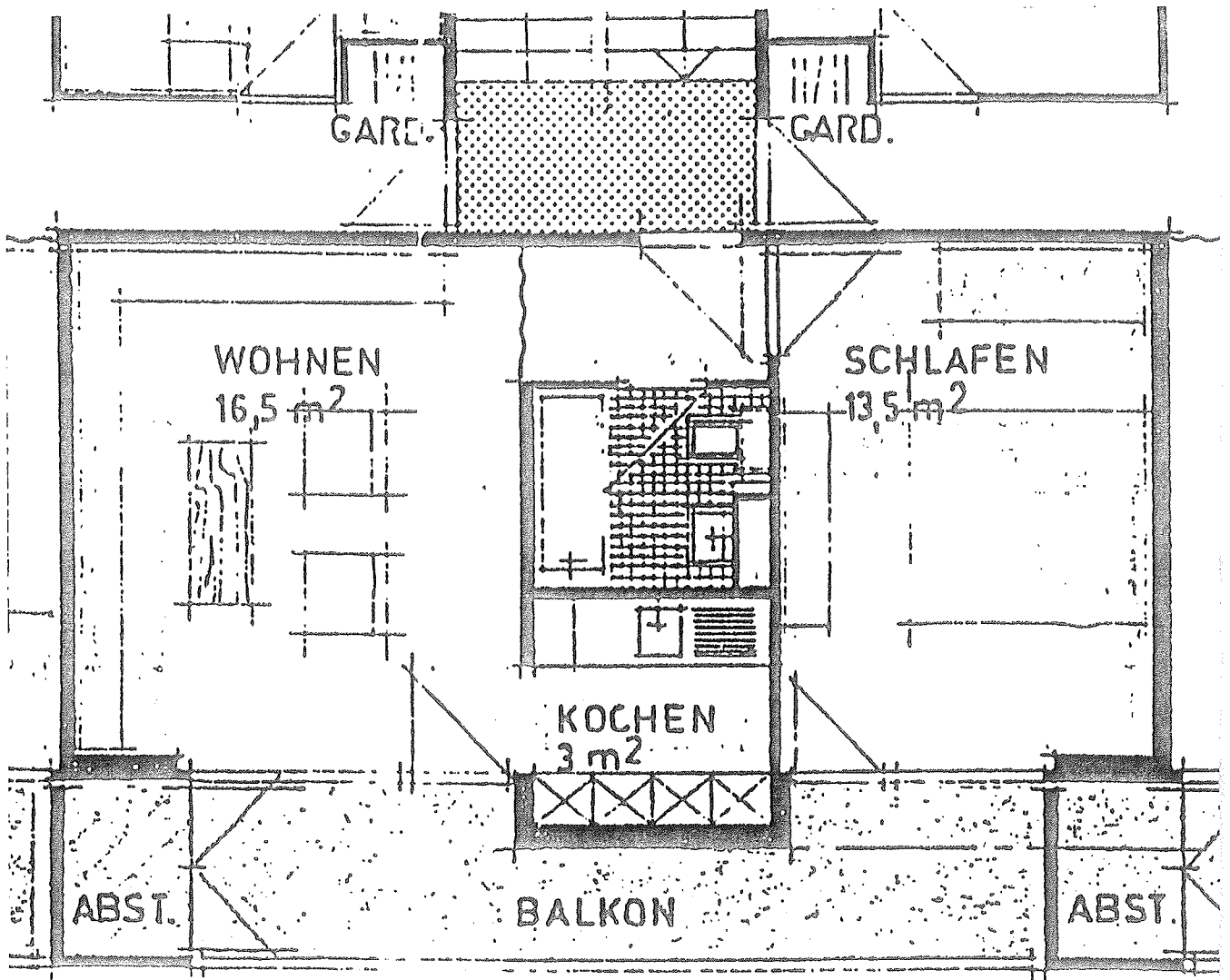
4.2 2 1/2-Zimmerwohnung
