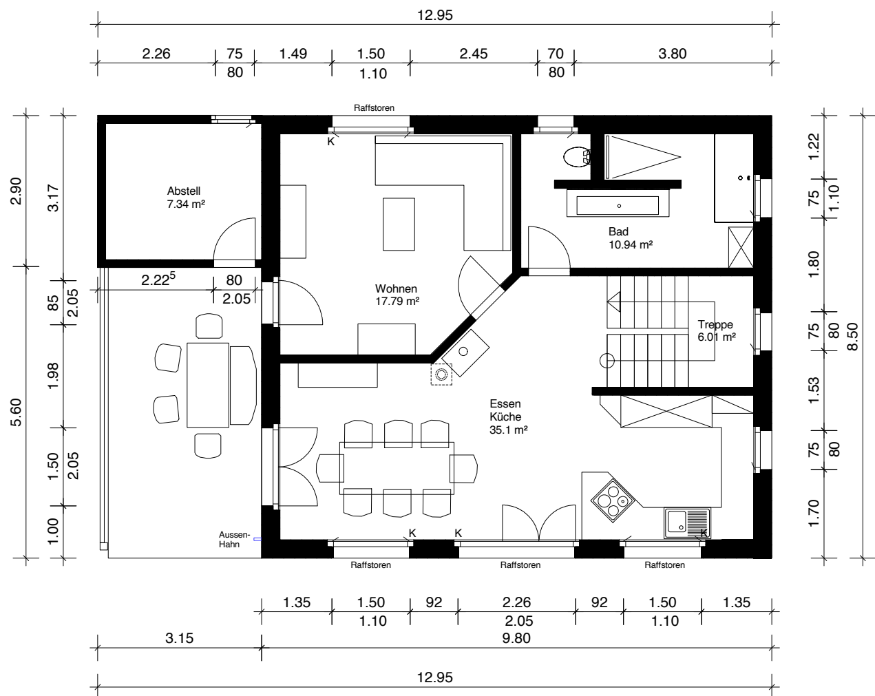
Erdbgeschoss
