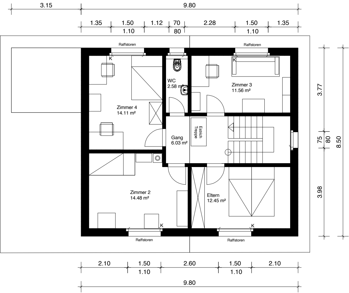
Obergeschoss
