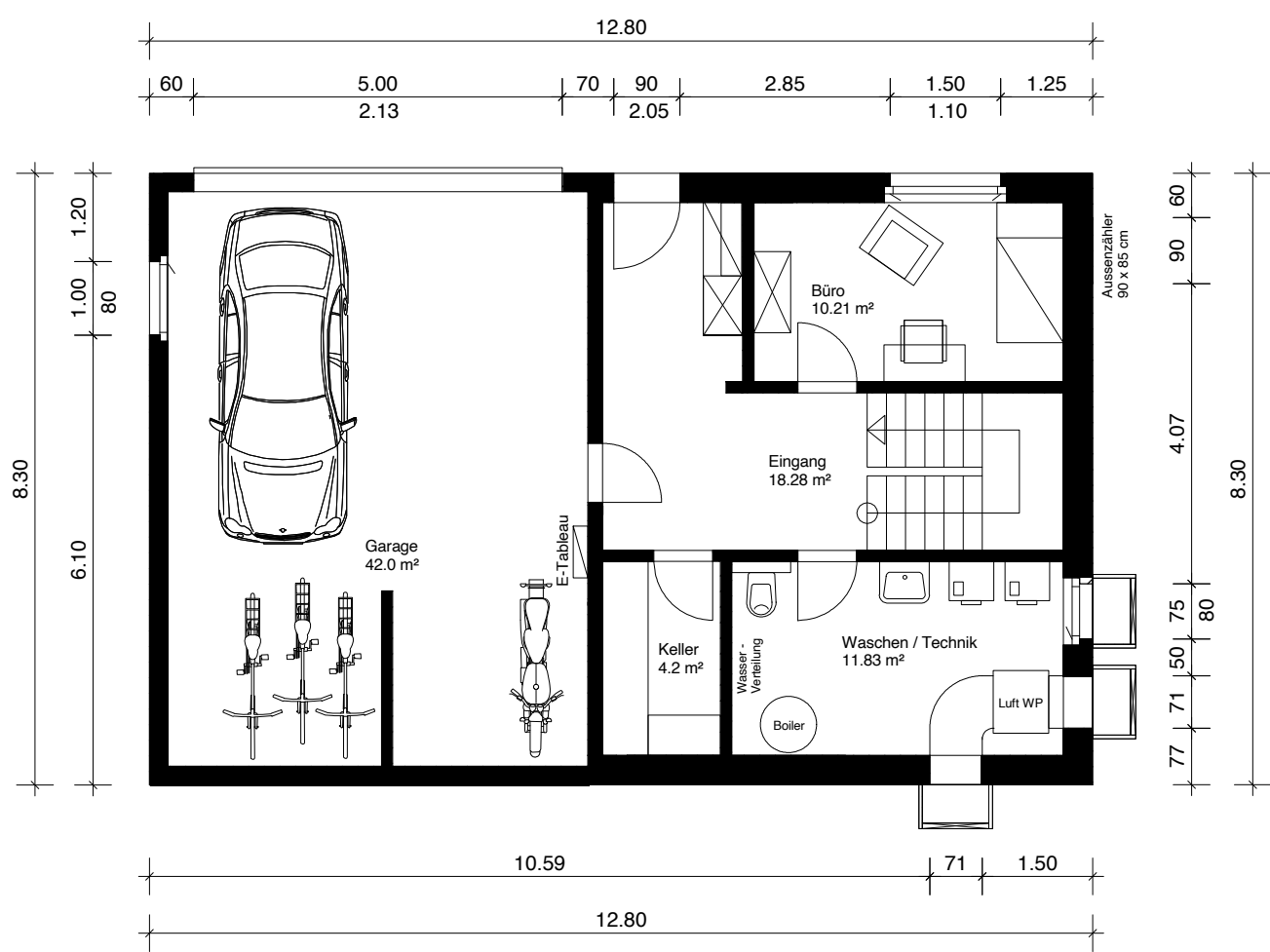
Kellergeschoss
