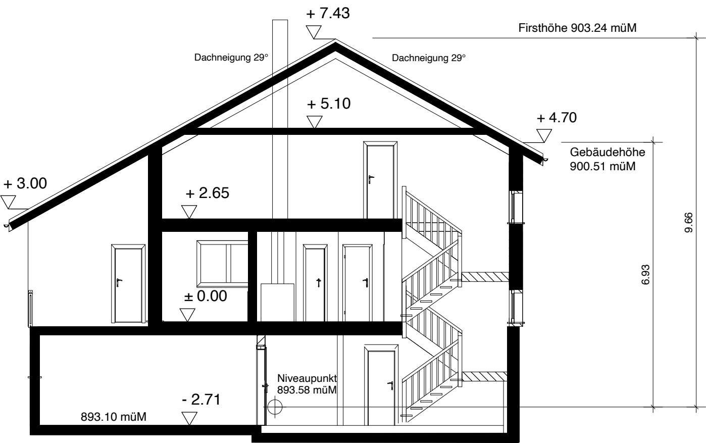
Schnitt
