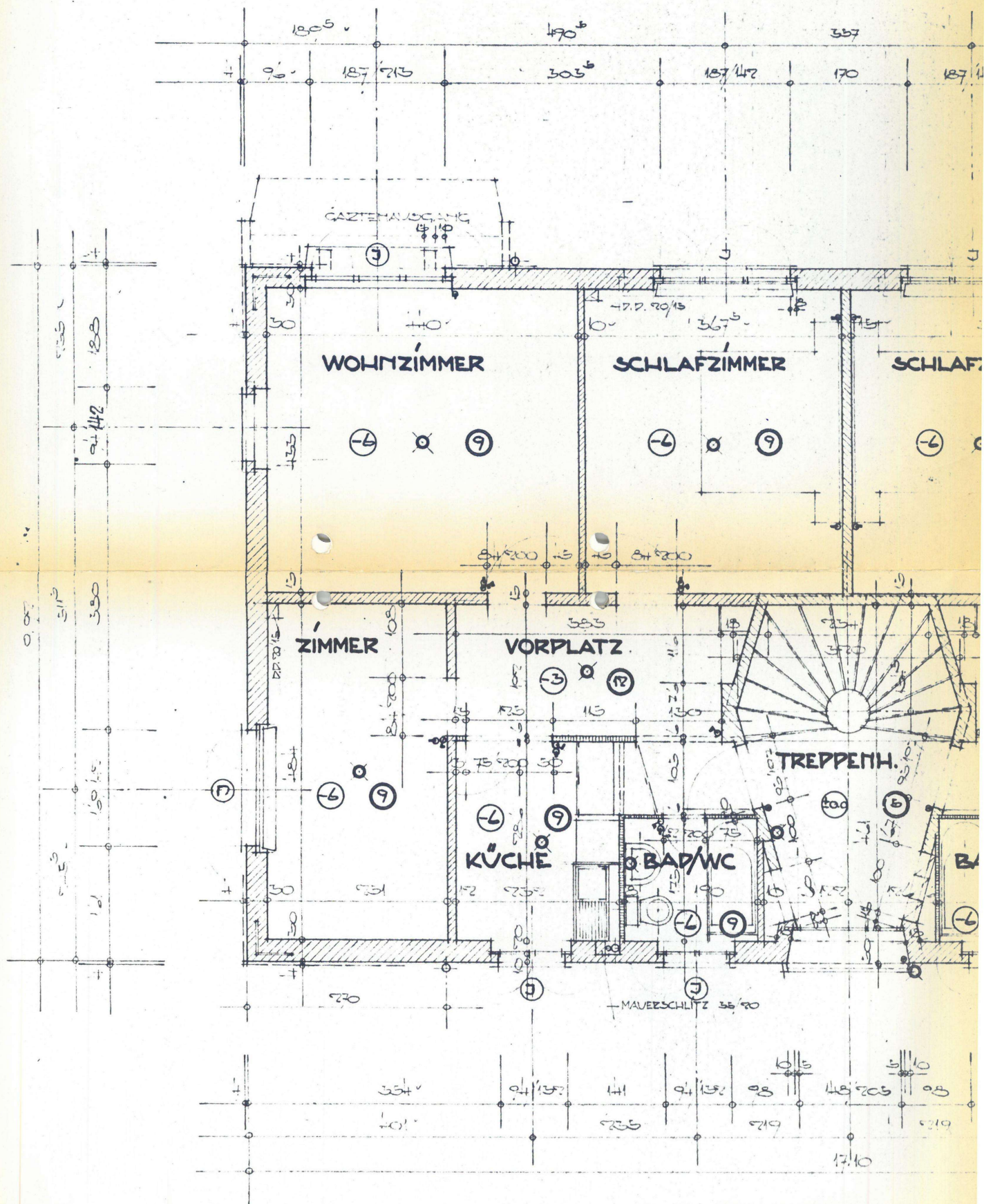
ERDGESCHOSS
