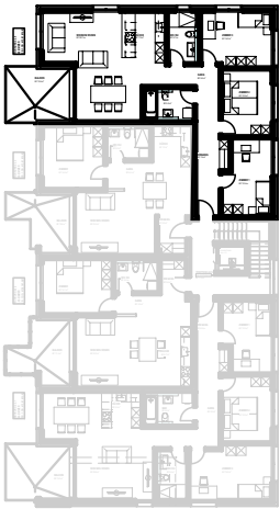
GESCHOSSÜBERSICHT
