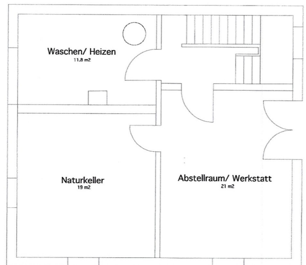
Grundriss Keller
