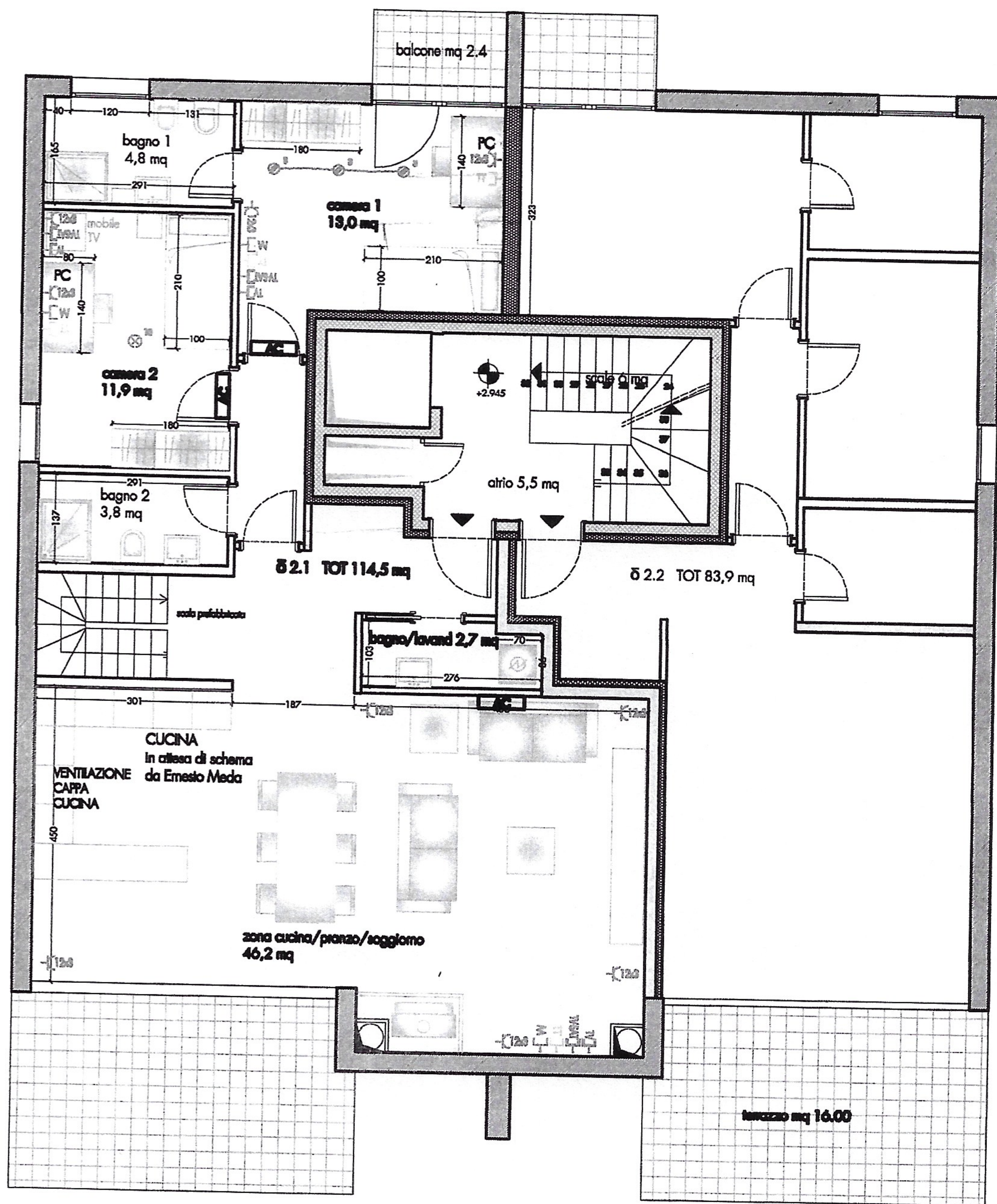
Edificio Delta - primo piano scala 1:100
