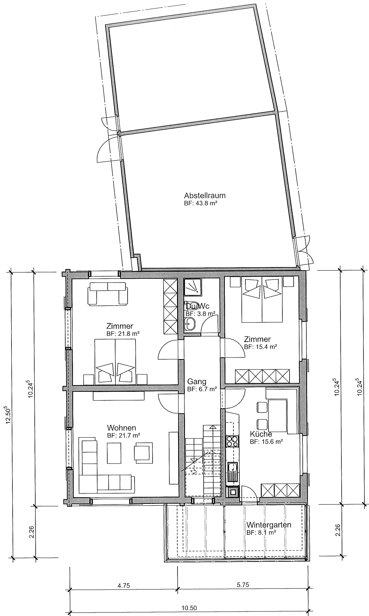
Erdgeschoss M. 1 : 100
