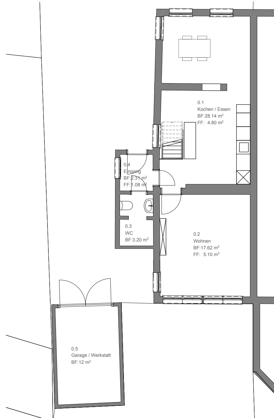
Erdgeschoss, mst. 1:100
