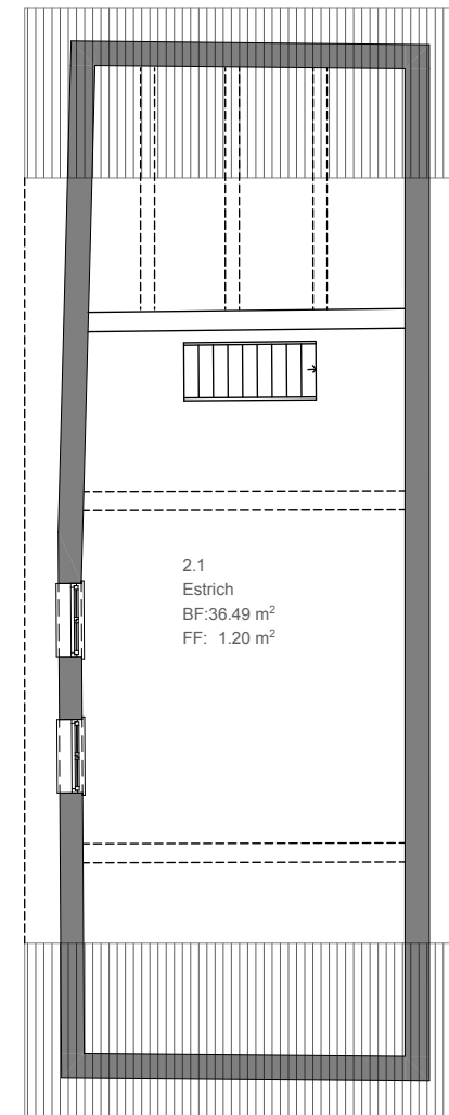
Dachgeschoss, mst. 1:100
