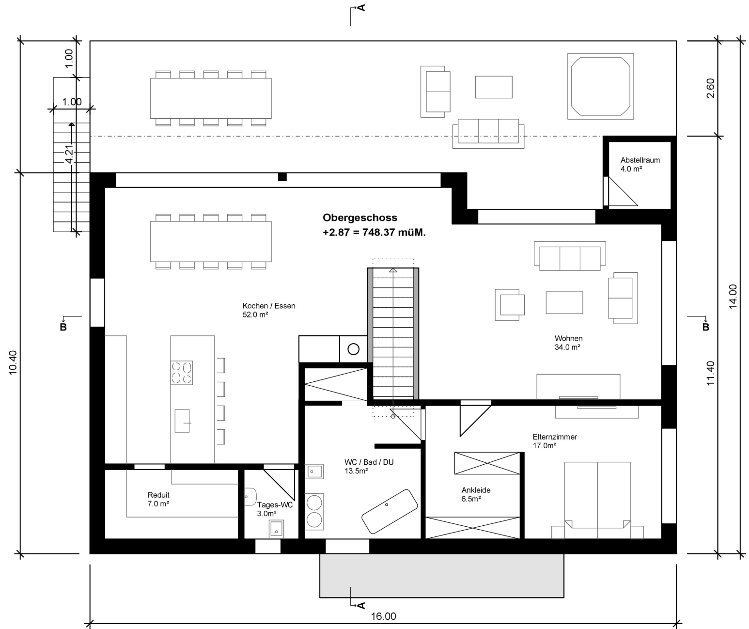
Einfamilienhaus - OBERGESCHOSS
