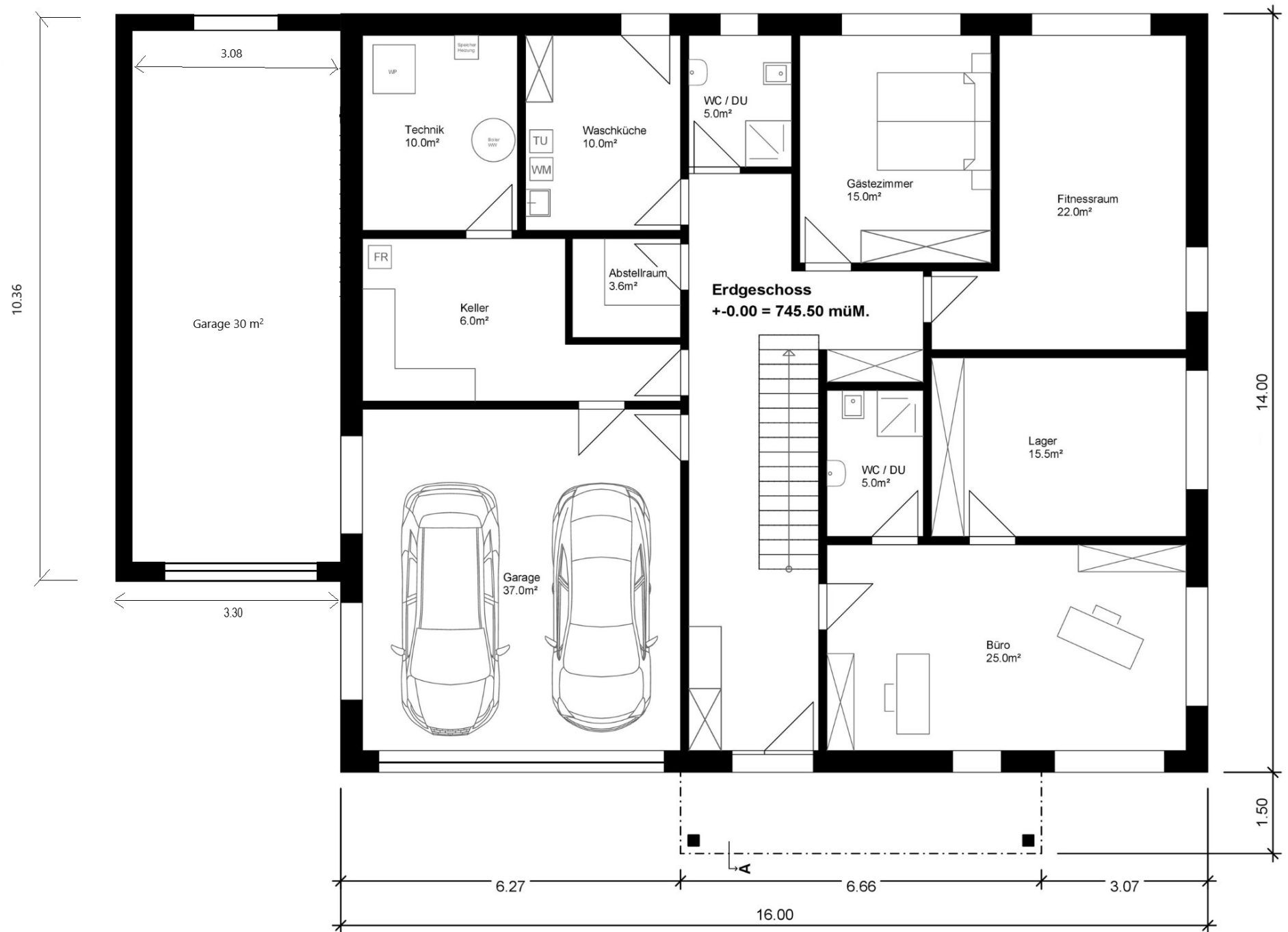
Einfamilienhaus - ERDGESCHOSS
