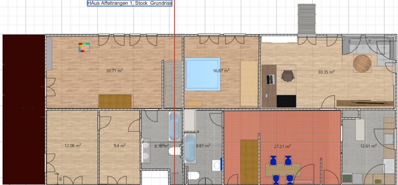
HAus Affeltrangen 1. Stock Grundriss
