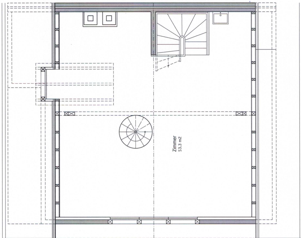
2. Obergeschoss 1 : 50 EFF Lützelbachweg 3 17.11.2016 mermet + burckhardt architekten ag hardstrasse 45 4020 basel
