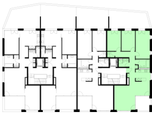
Geschossübersicht
