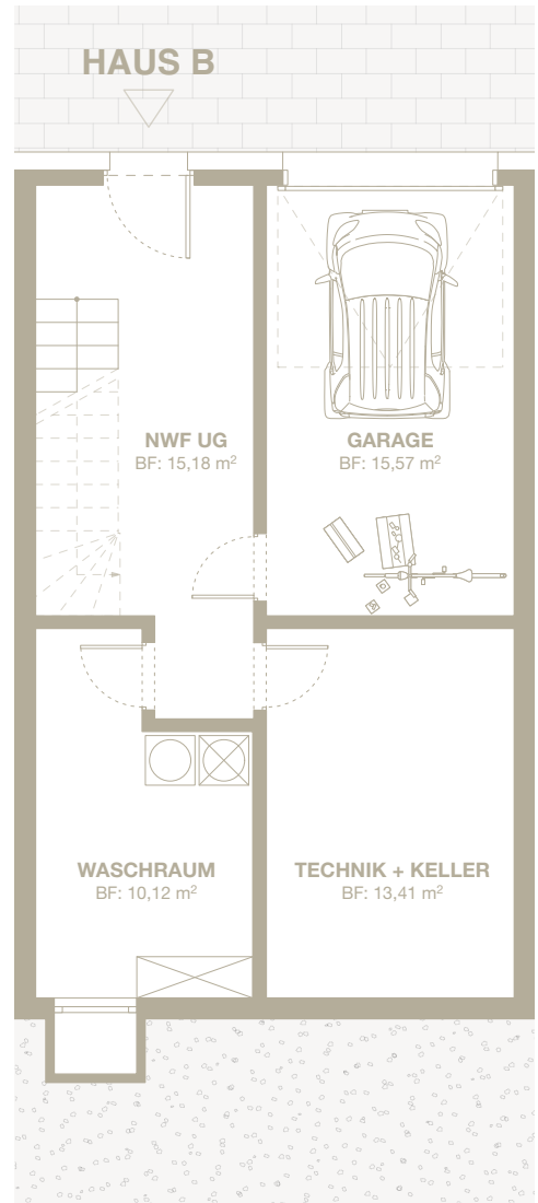
UNTERGESCHOSS
