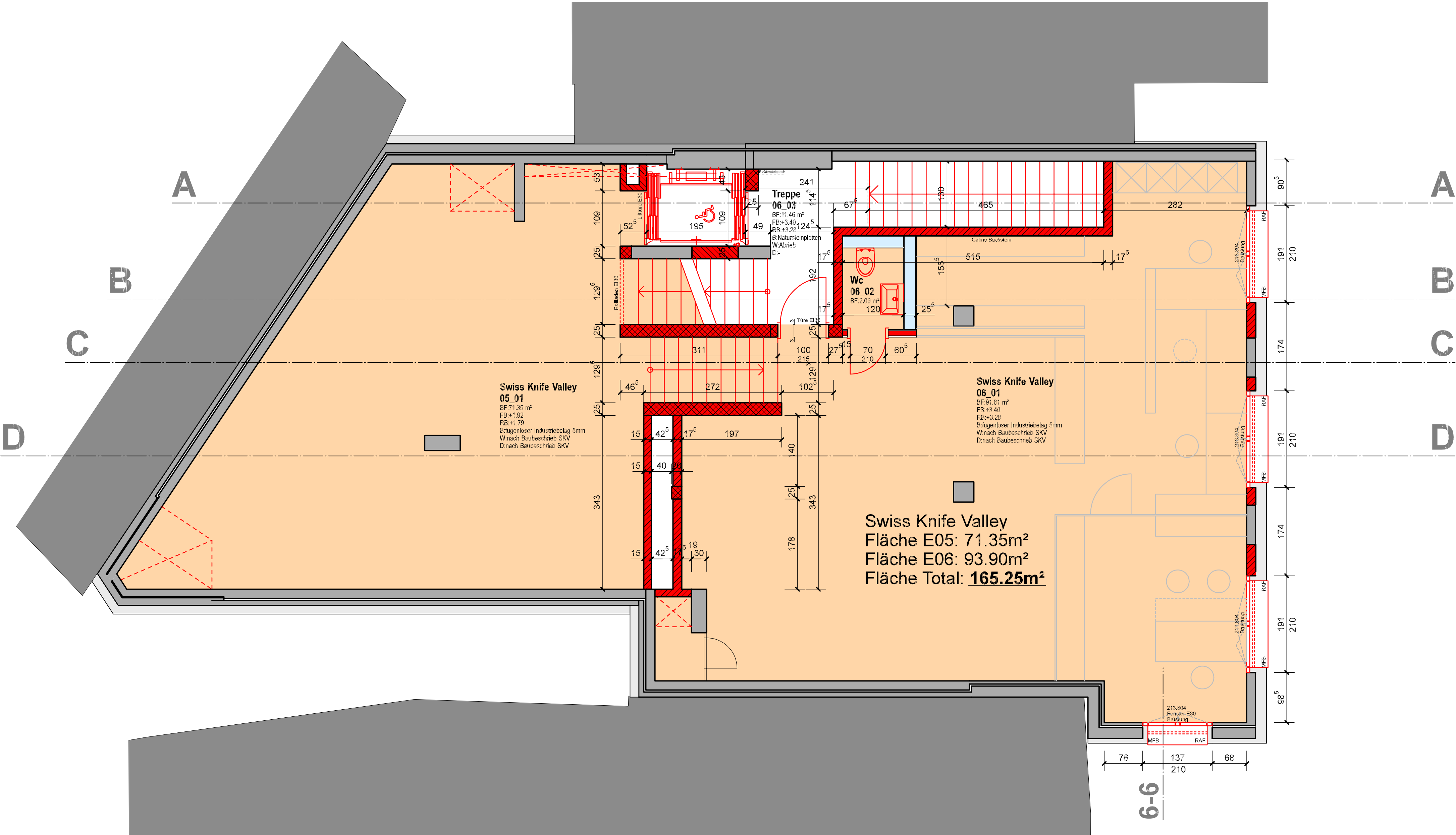
1. Obergeschoss Ebene 05
