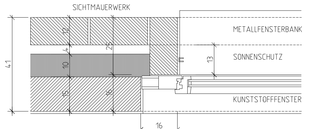
ANSCHLAGDETAIL 1:10 (AUCH SPIEGELBILDICH)
