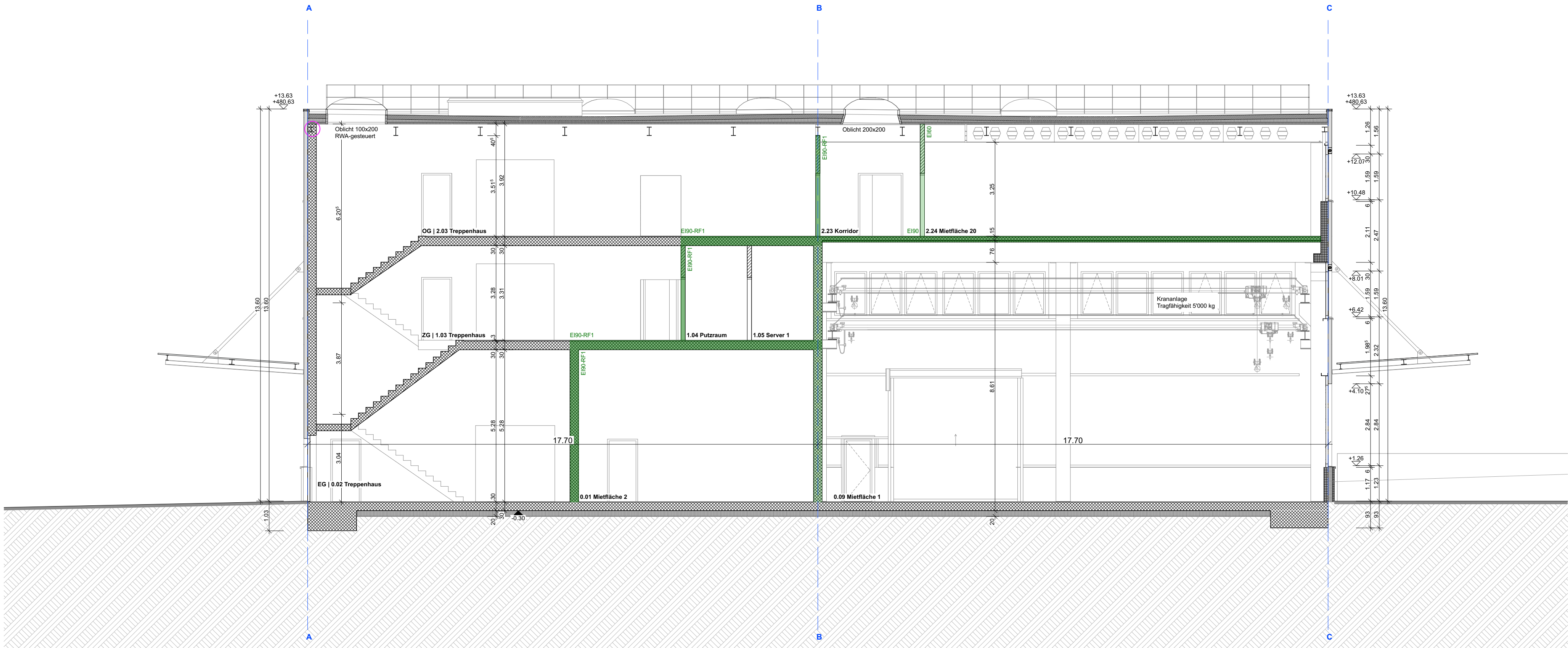
Querschnitt 2
