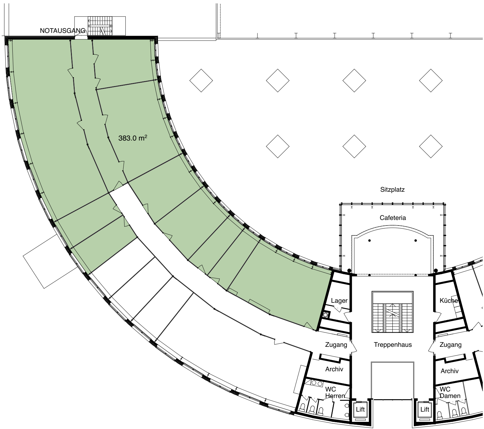
3.0 Grundriss 3.OG
