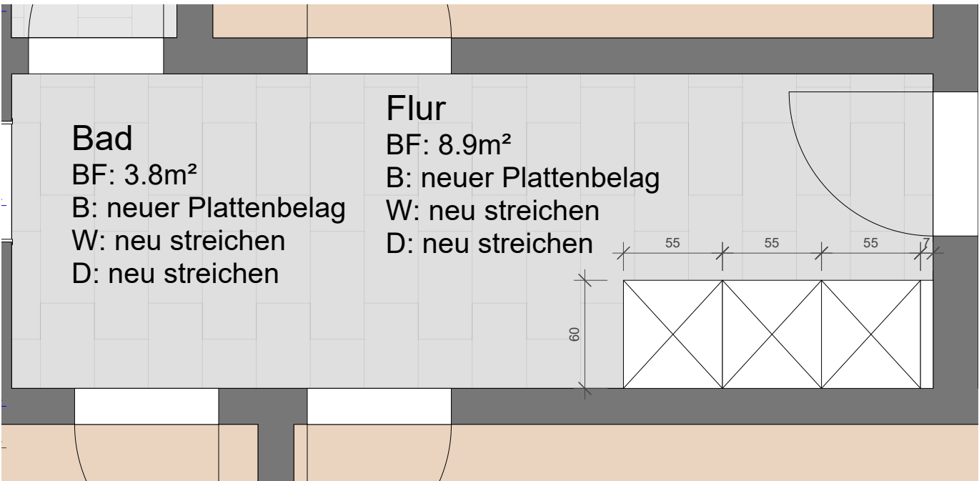
Grundriss
