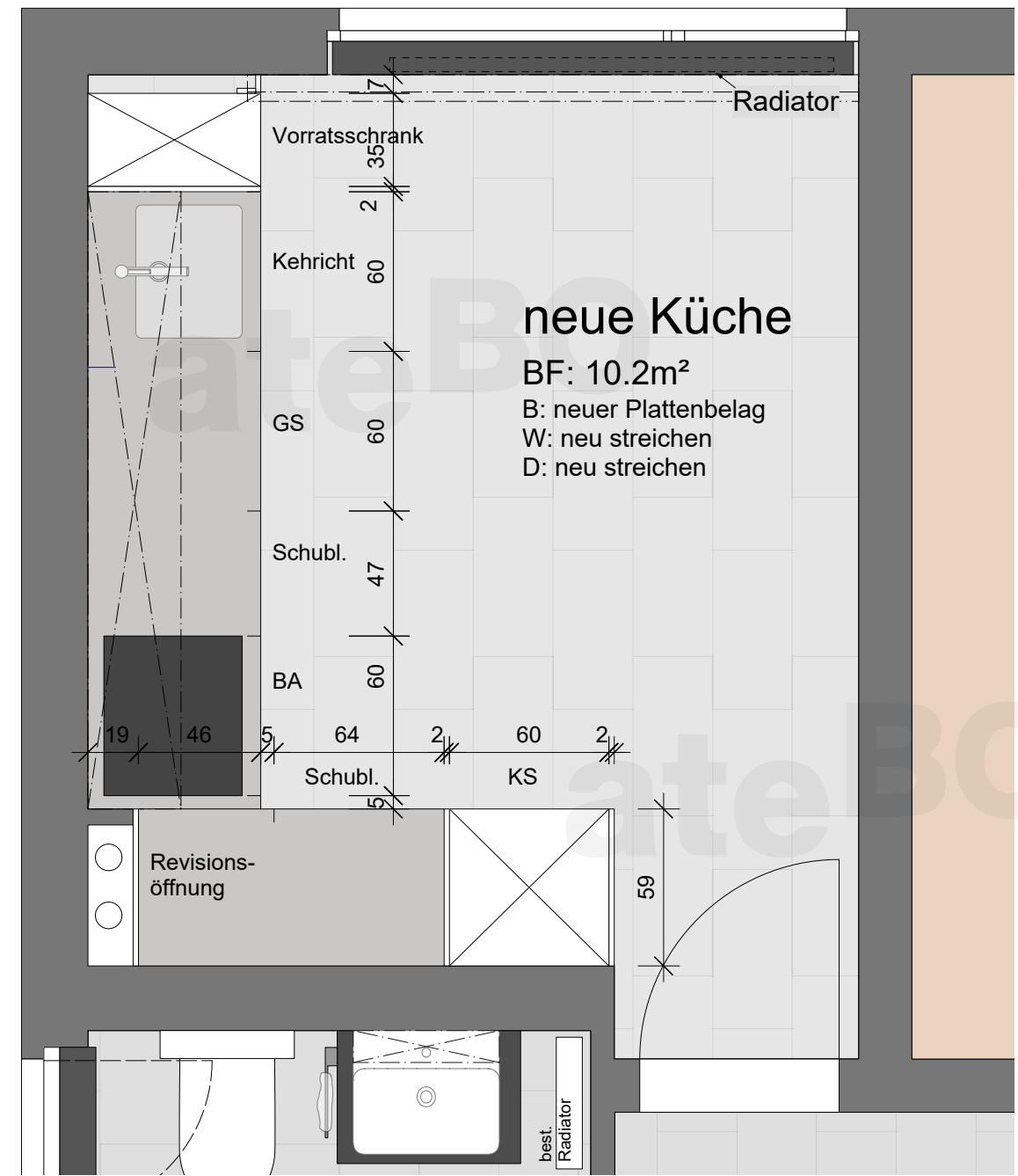
Grundriss
