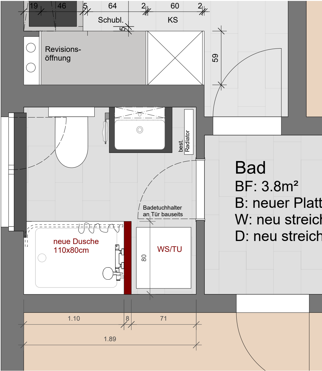
Grundriss
