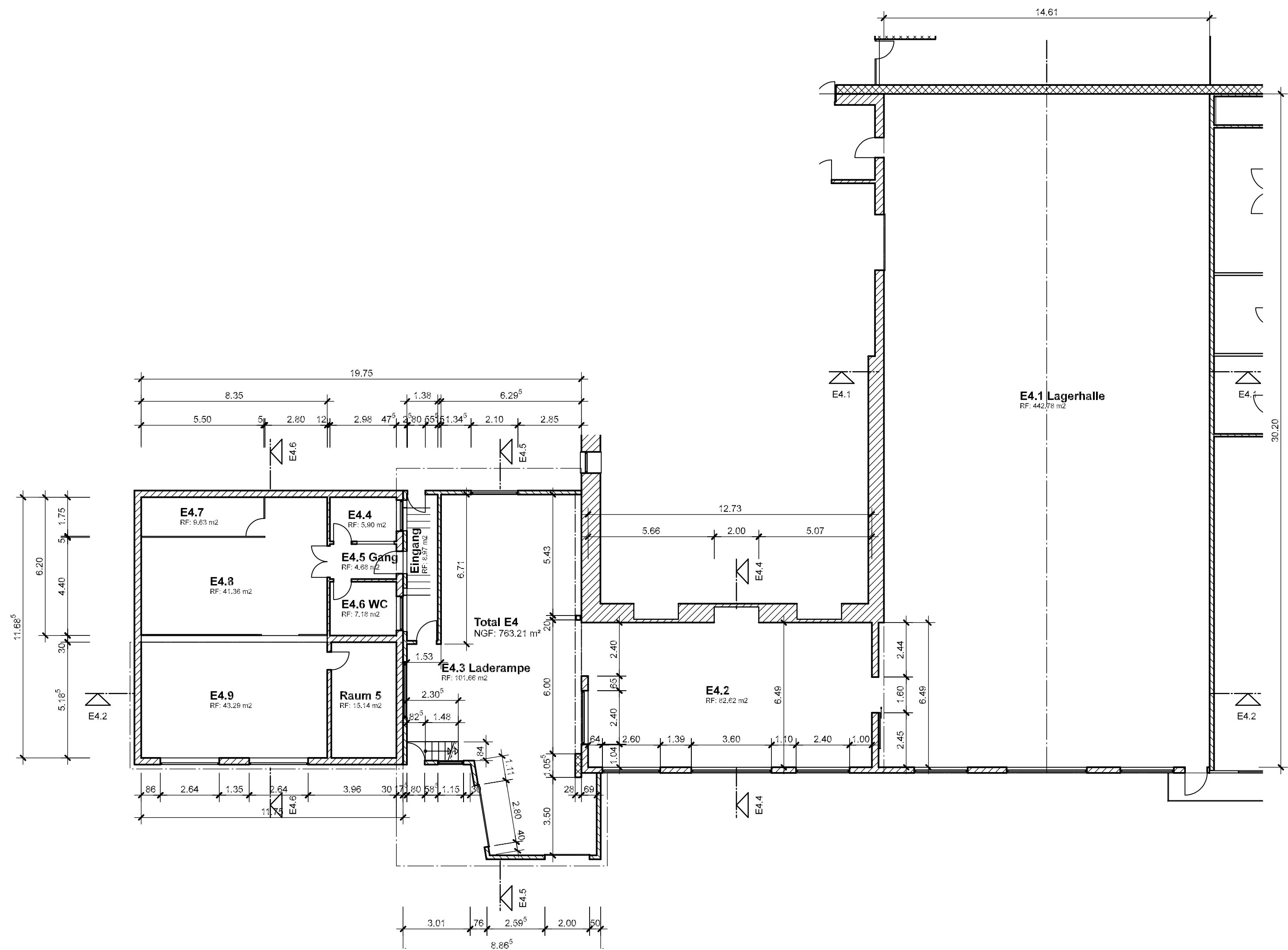
Grundriss E4 1:150
