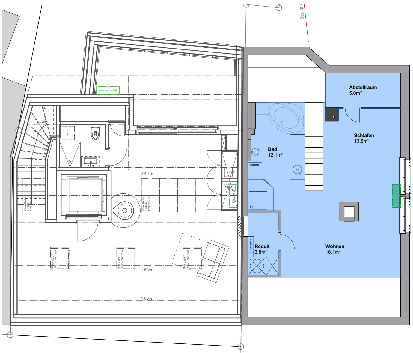
Grundriss Dachgeschoss Wohnung Zürichstrasse 3 | 50.8 m²
