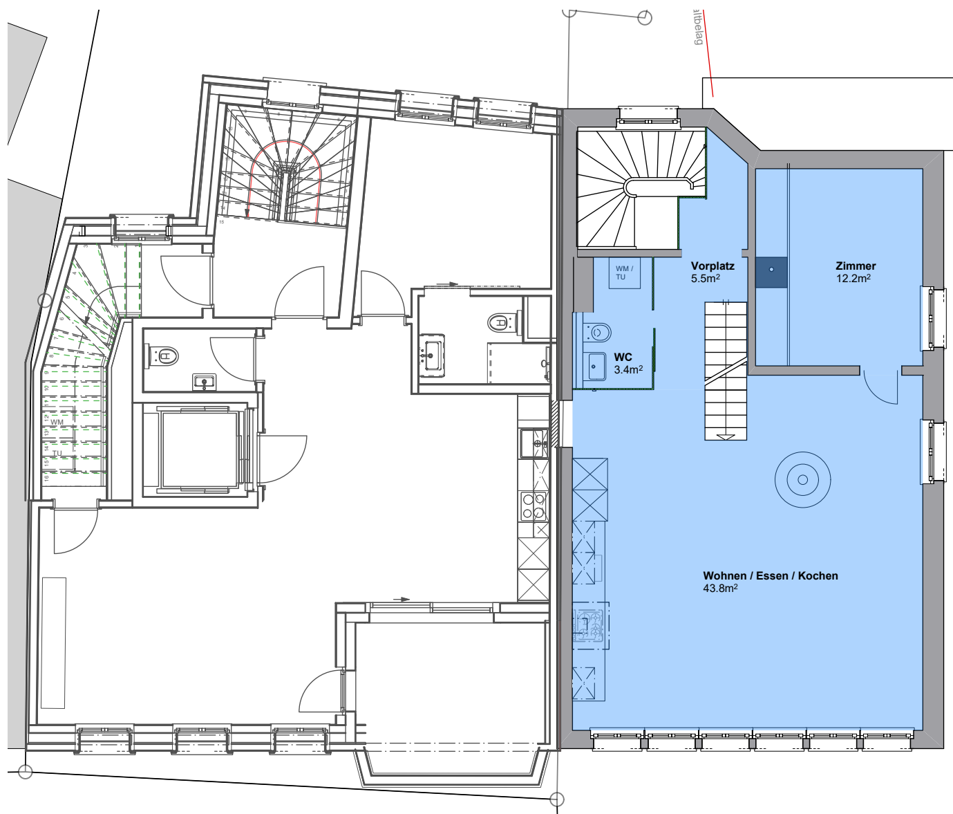
Grundriss 2. Obergeschoss Wohnung Zürichstrasse 3 | 65.0 m²
