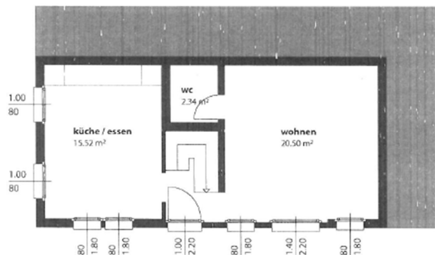
singenbergstrasse 6, 9000 st. gallen erdgeschoss 1:100
