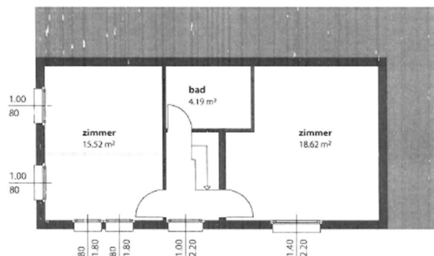
singenbergstrasse 6, 9000 st. gallen obergeschoss 1:100
