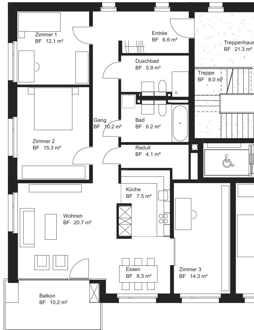
Typ A / Wohnung 1 und 5 4 1/2 Zi-Whg 111.2m 2
